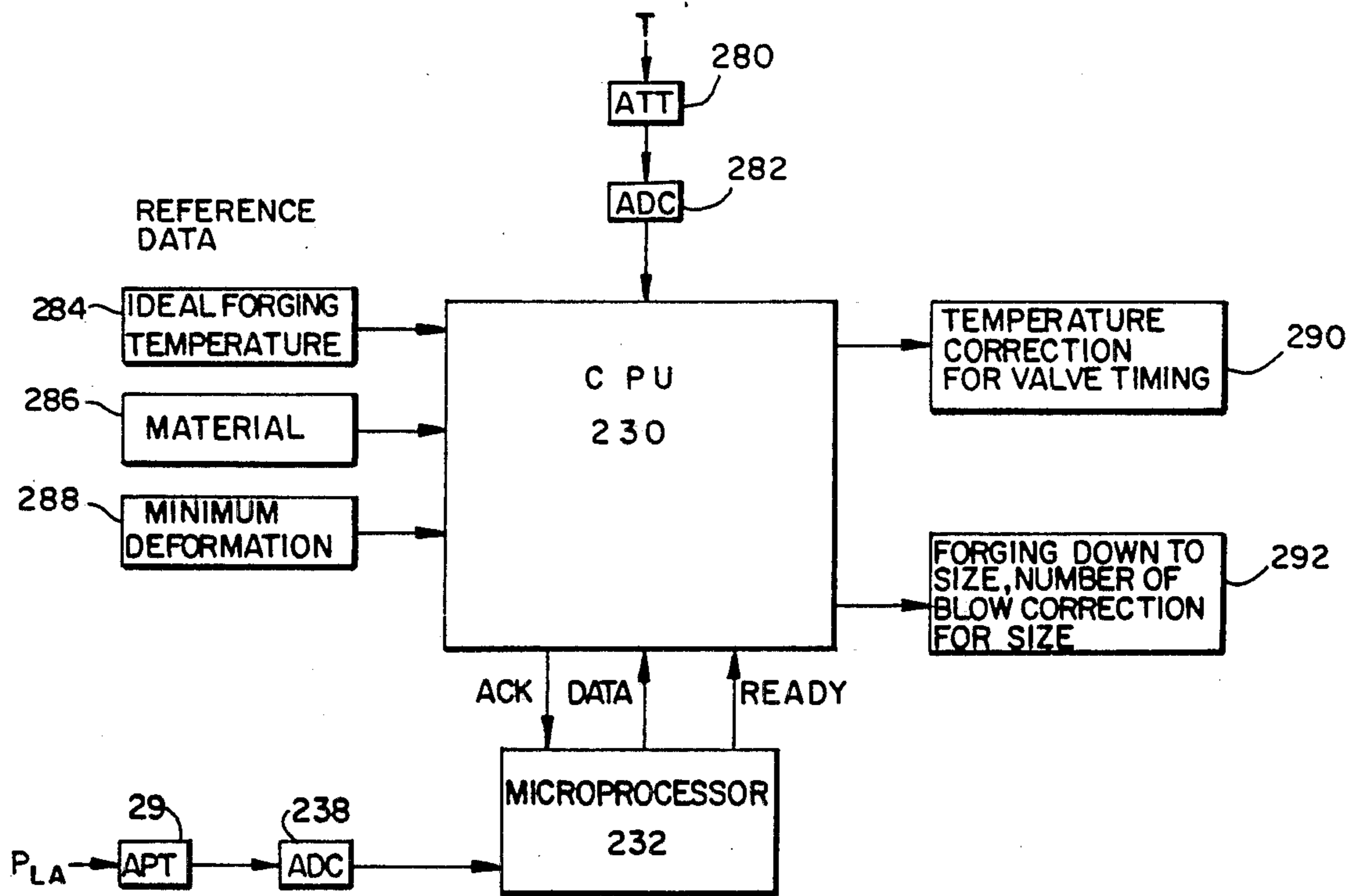
FIG. 9d
