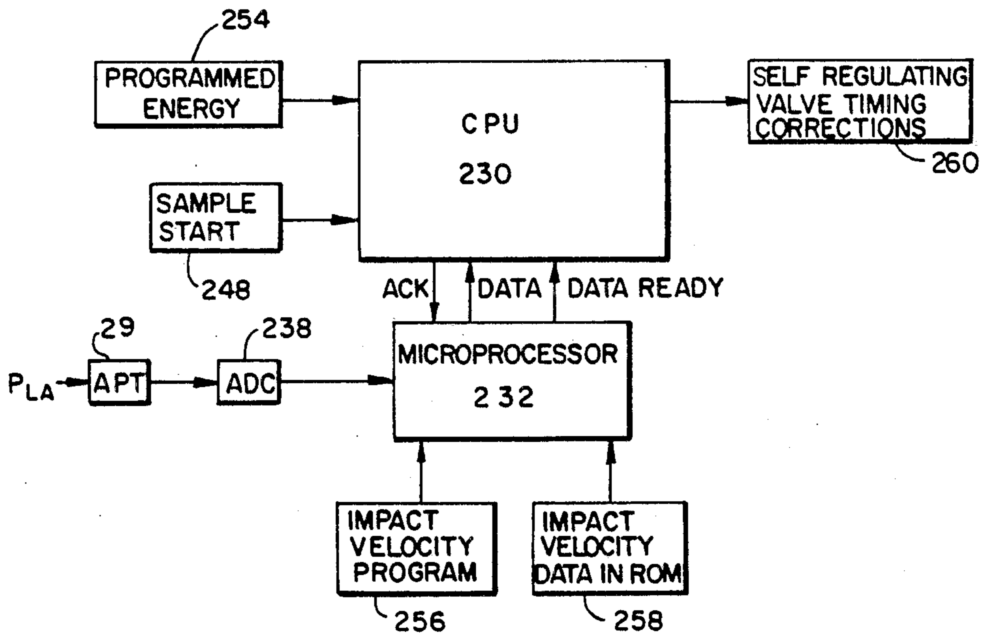
FIG. 9b
