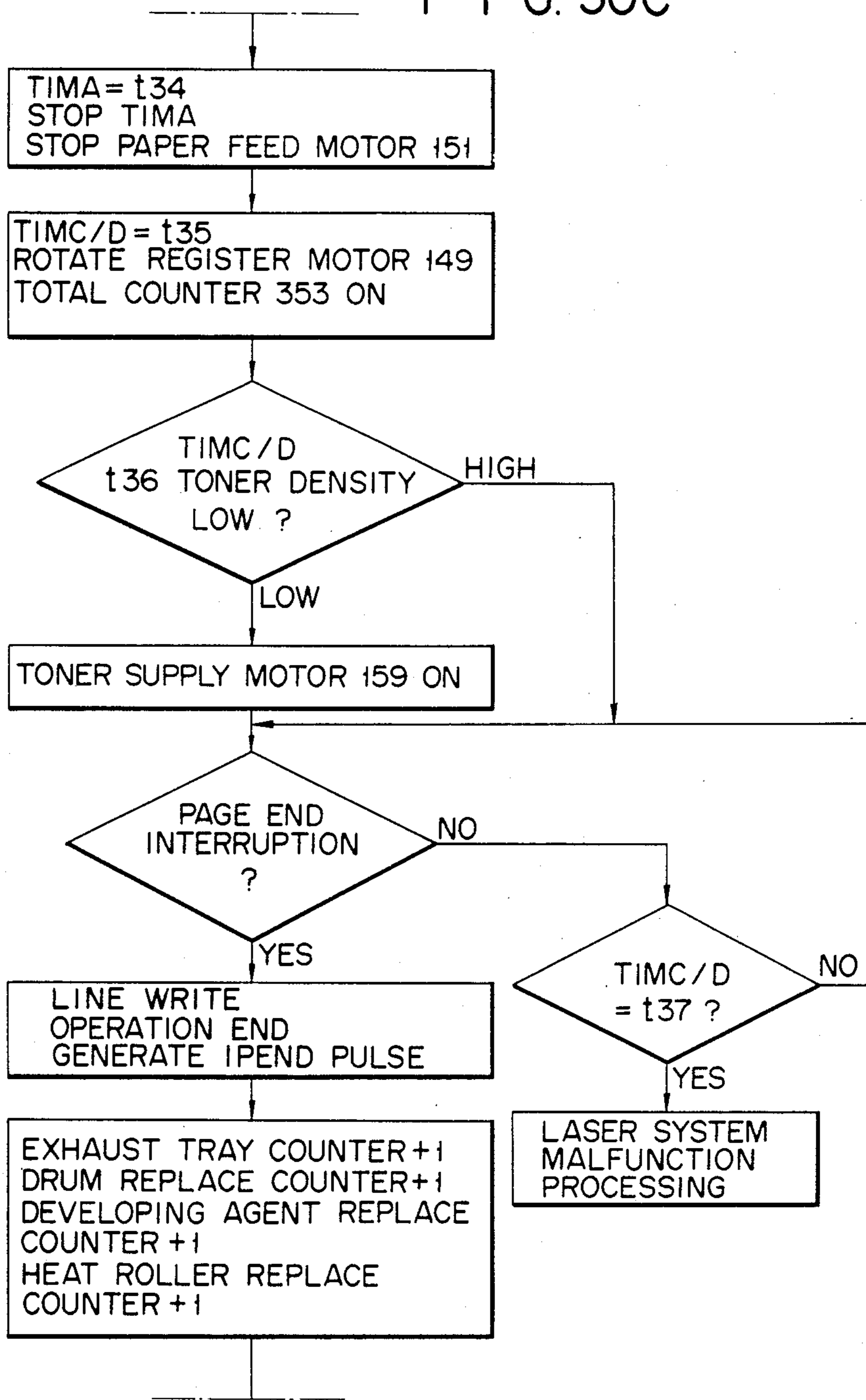
F I G. 50C
