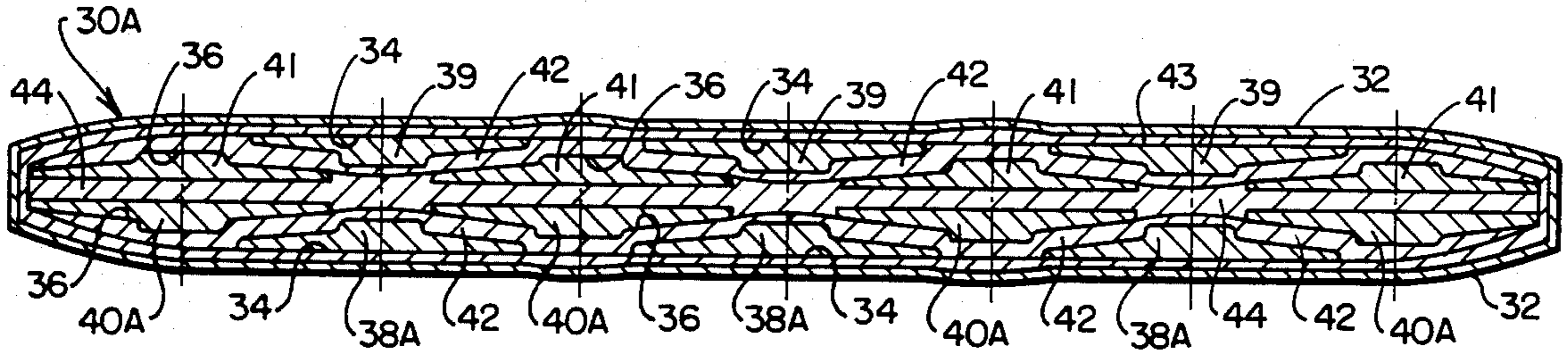
FIG. 7-A
