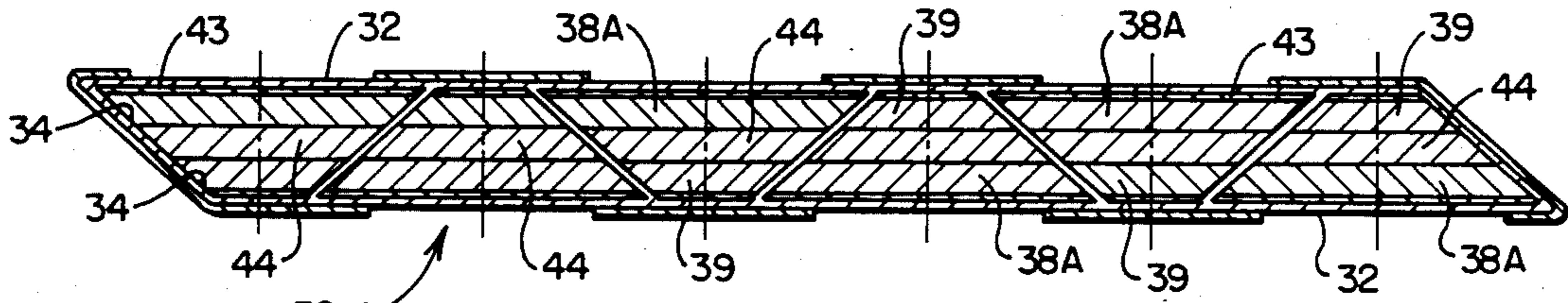
FIG. 16
