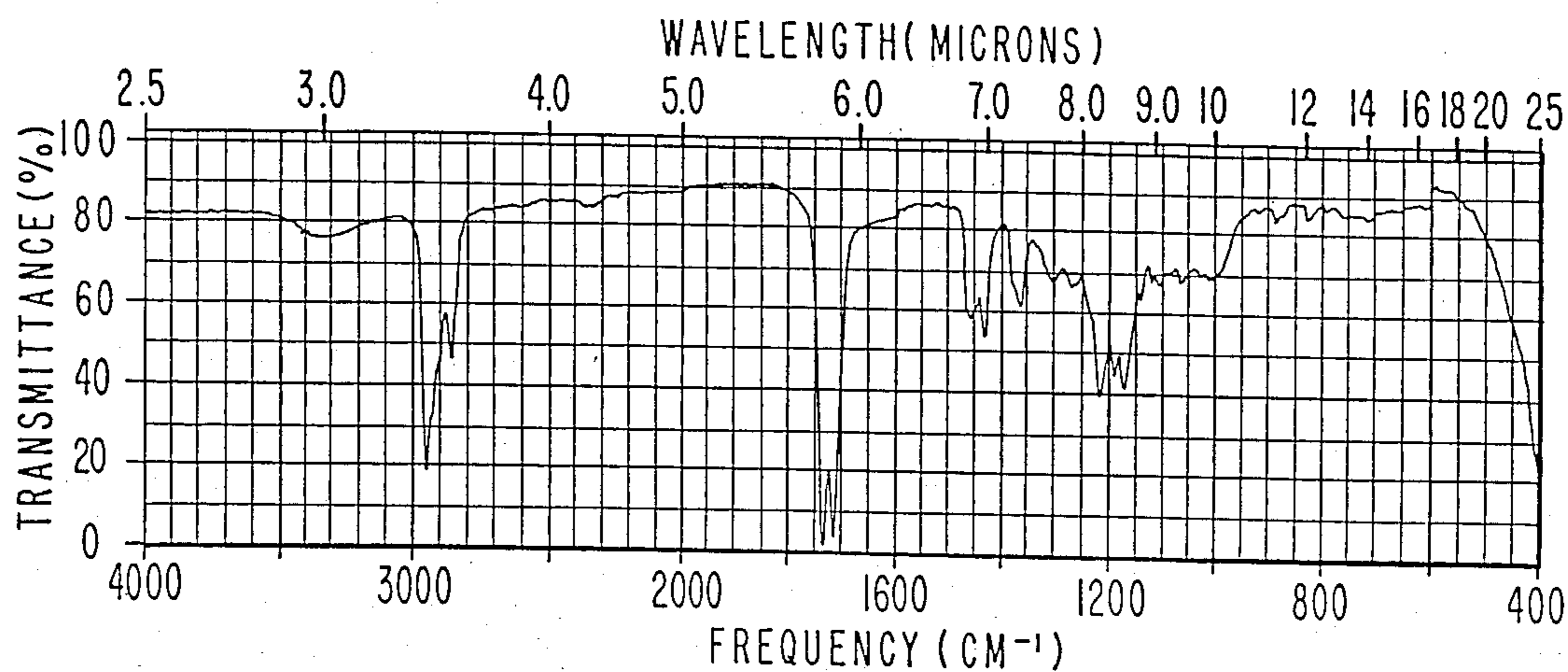
IR SPECTRUM FOR EXAMPLE X.
