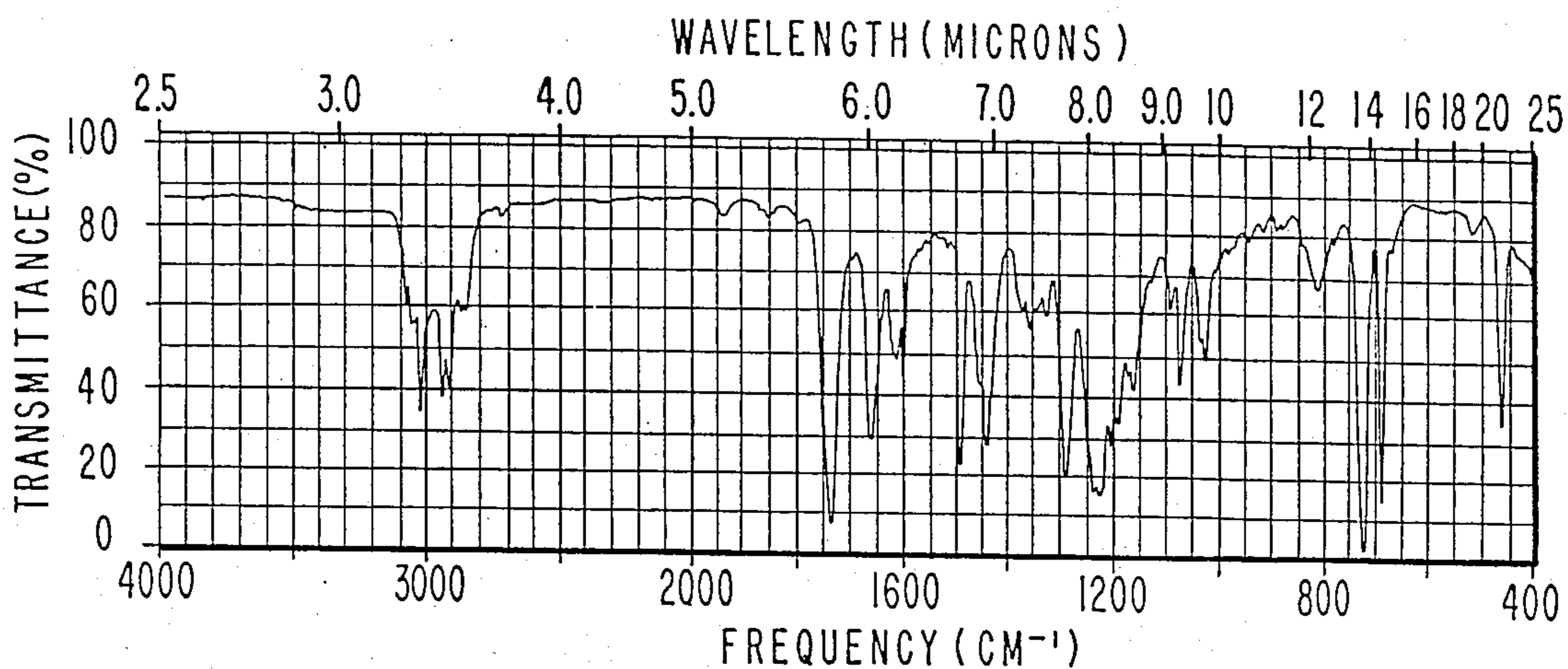
IR SPECTRUM FOR EXAMPLE XI(A).
