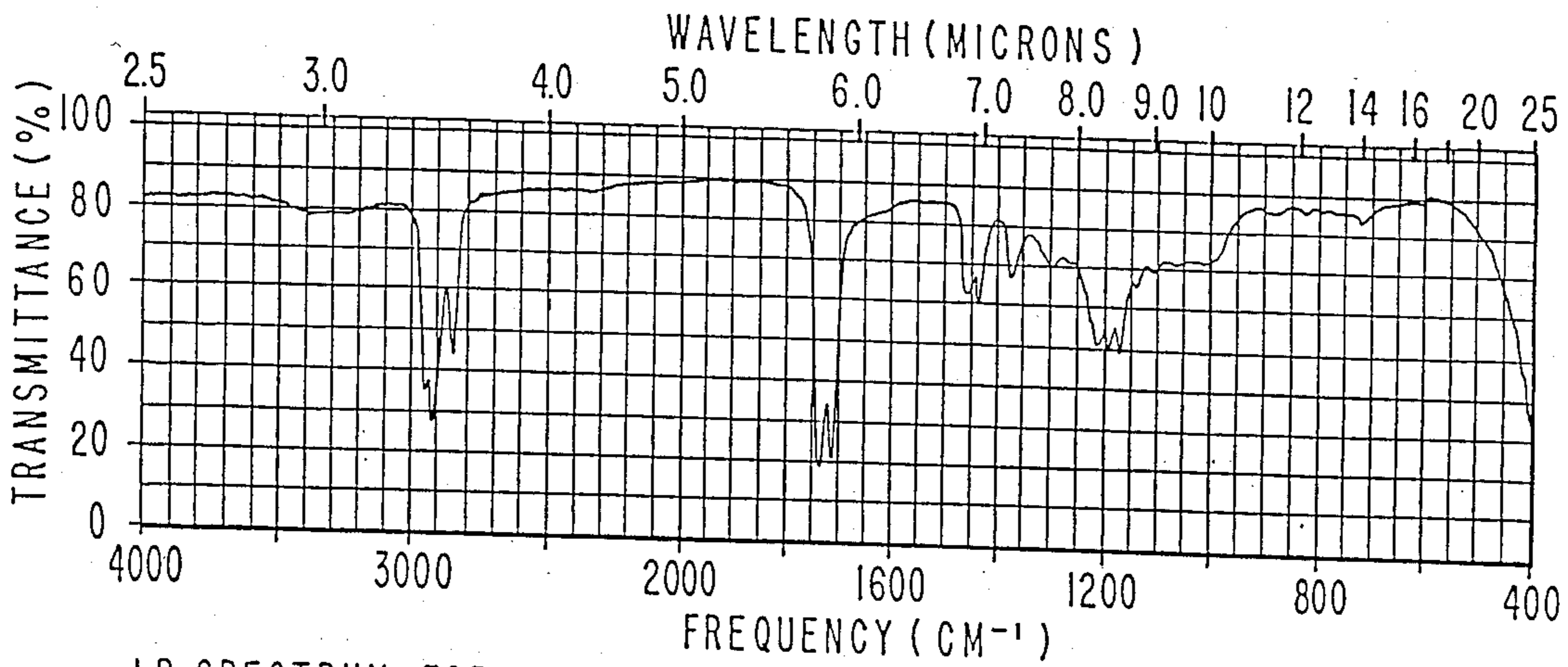
IR SPECTRUM FOR EXAMPLE VI.
