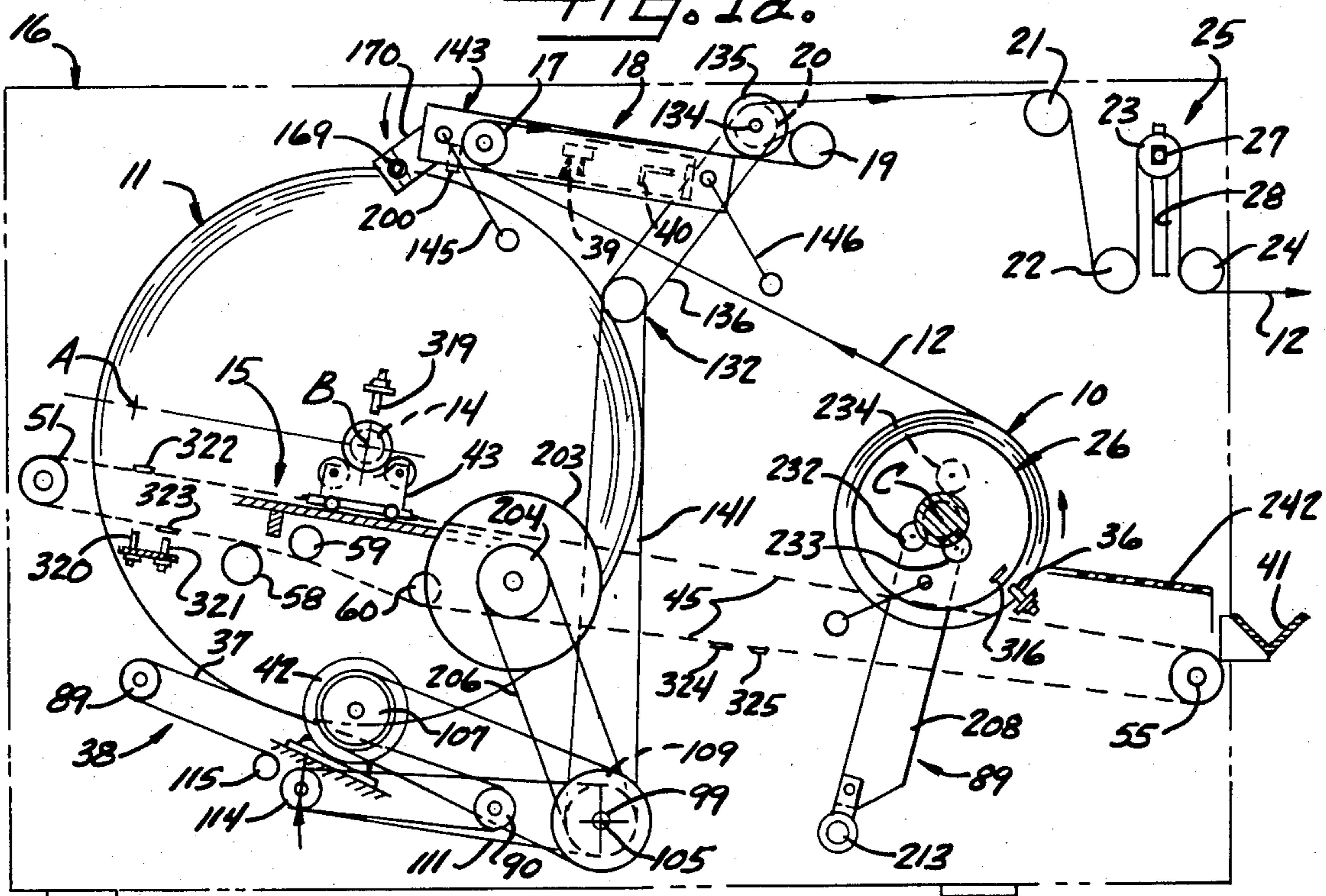
FIG. 16.
