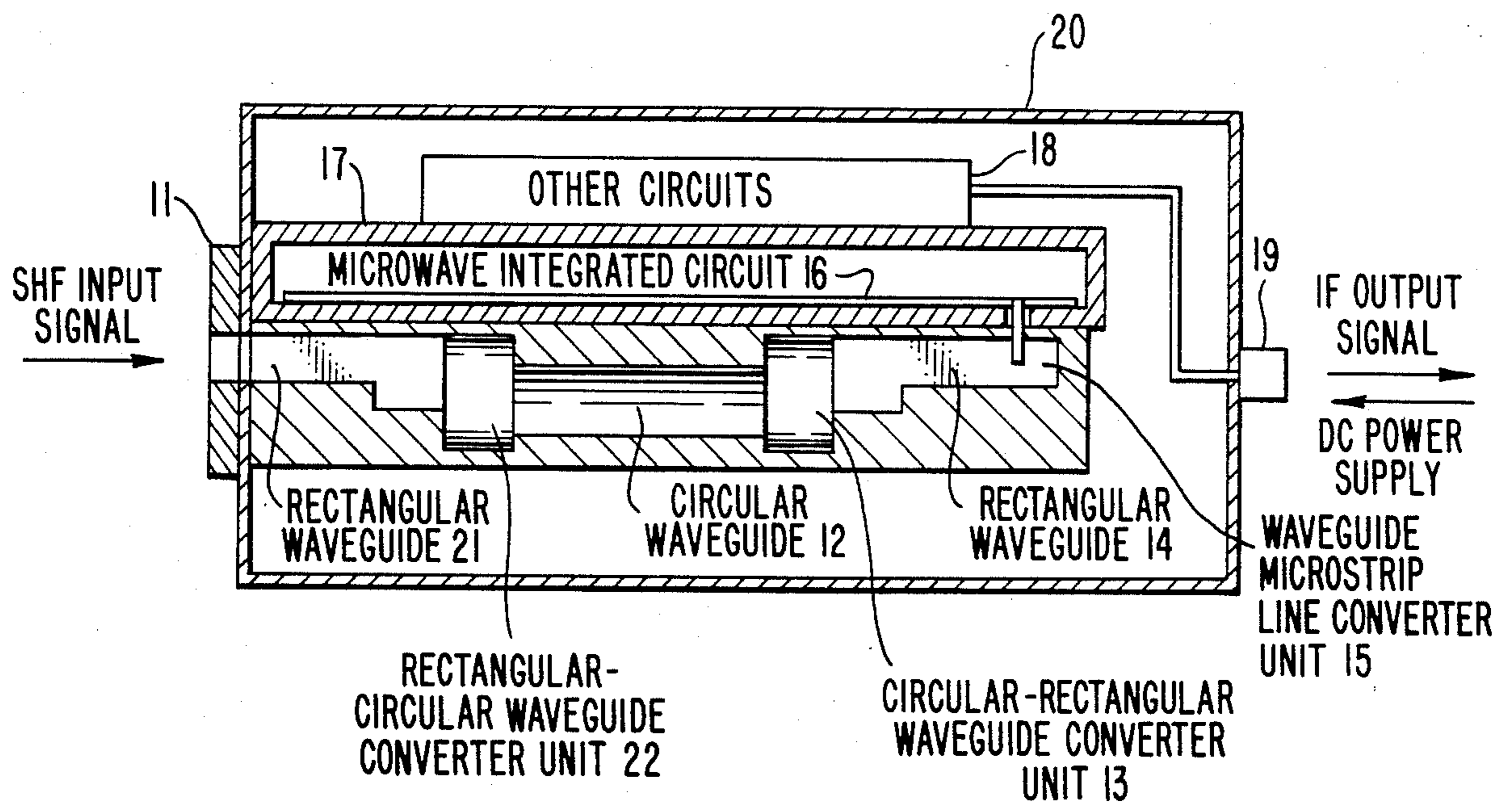
FIG. 8.
