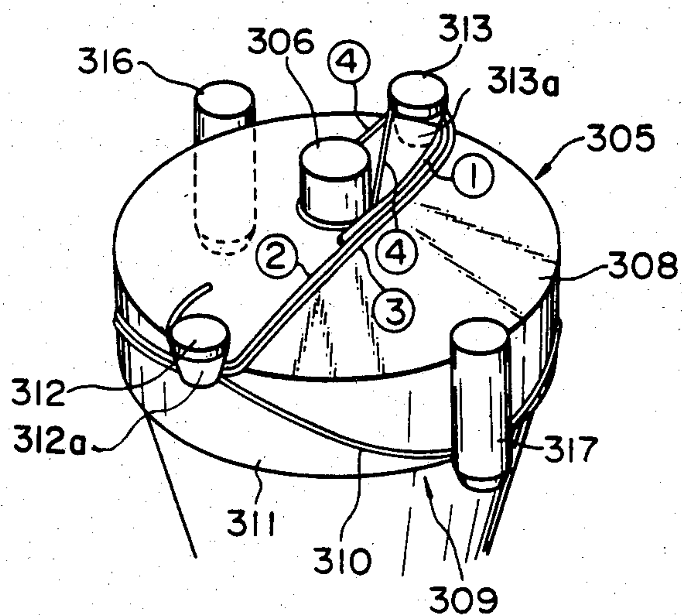
FIG. 25B
