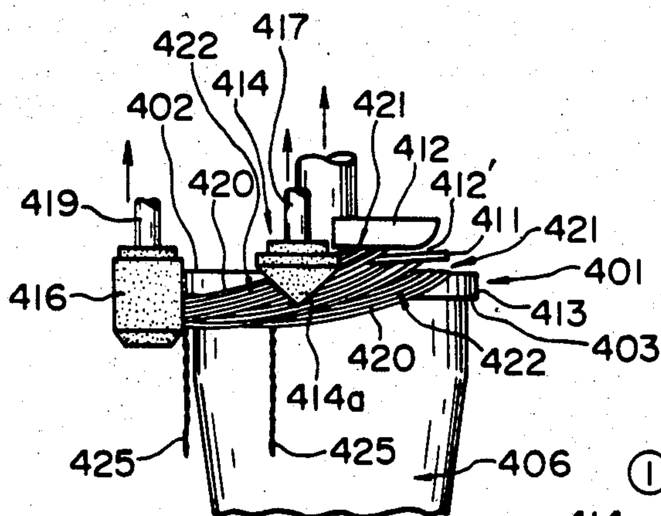
FIG. 31
