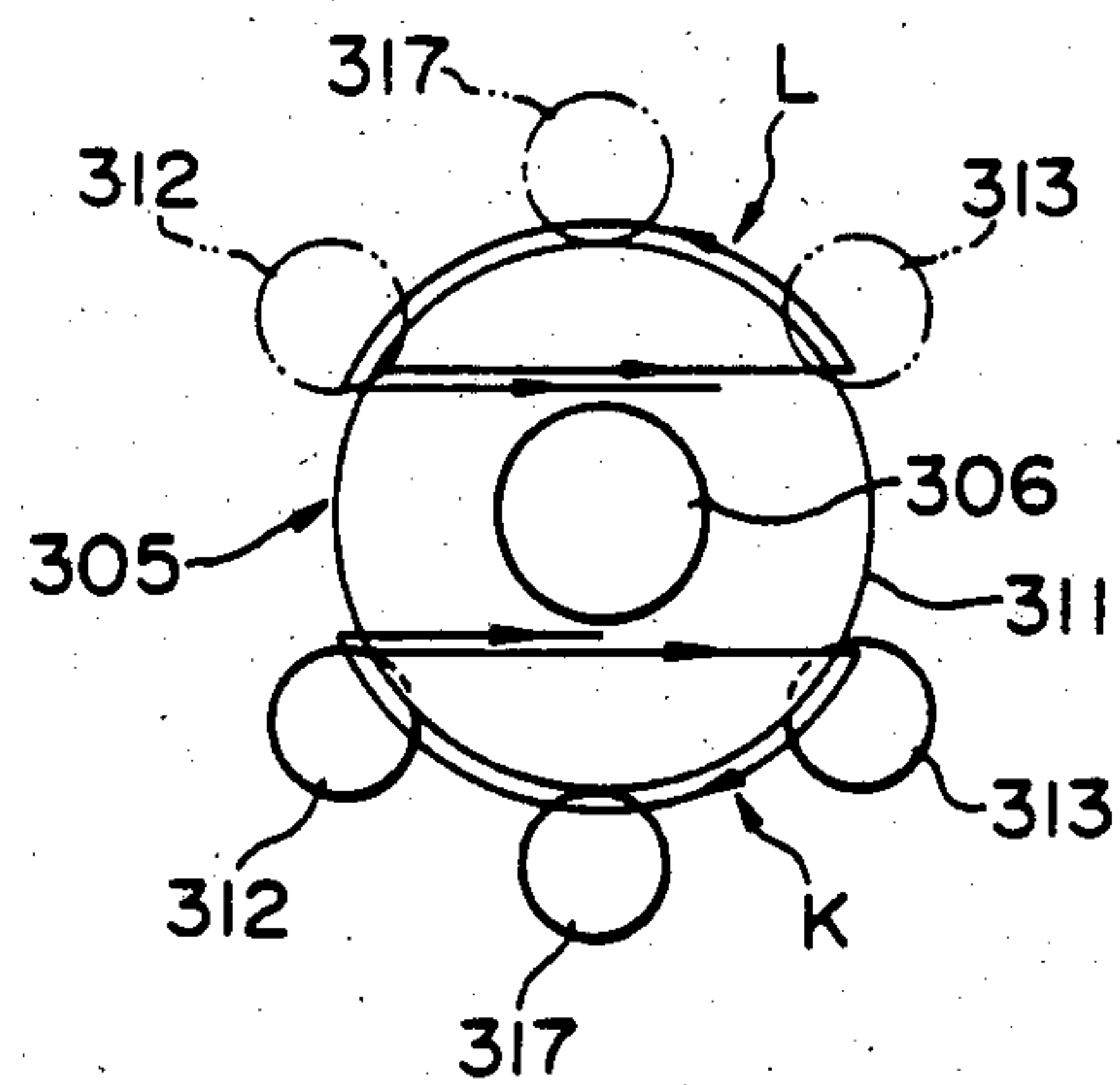
FIG. 28
