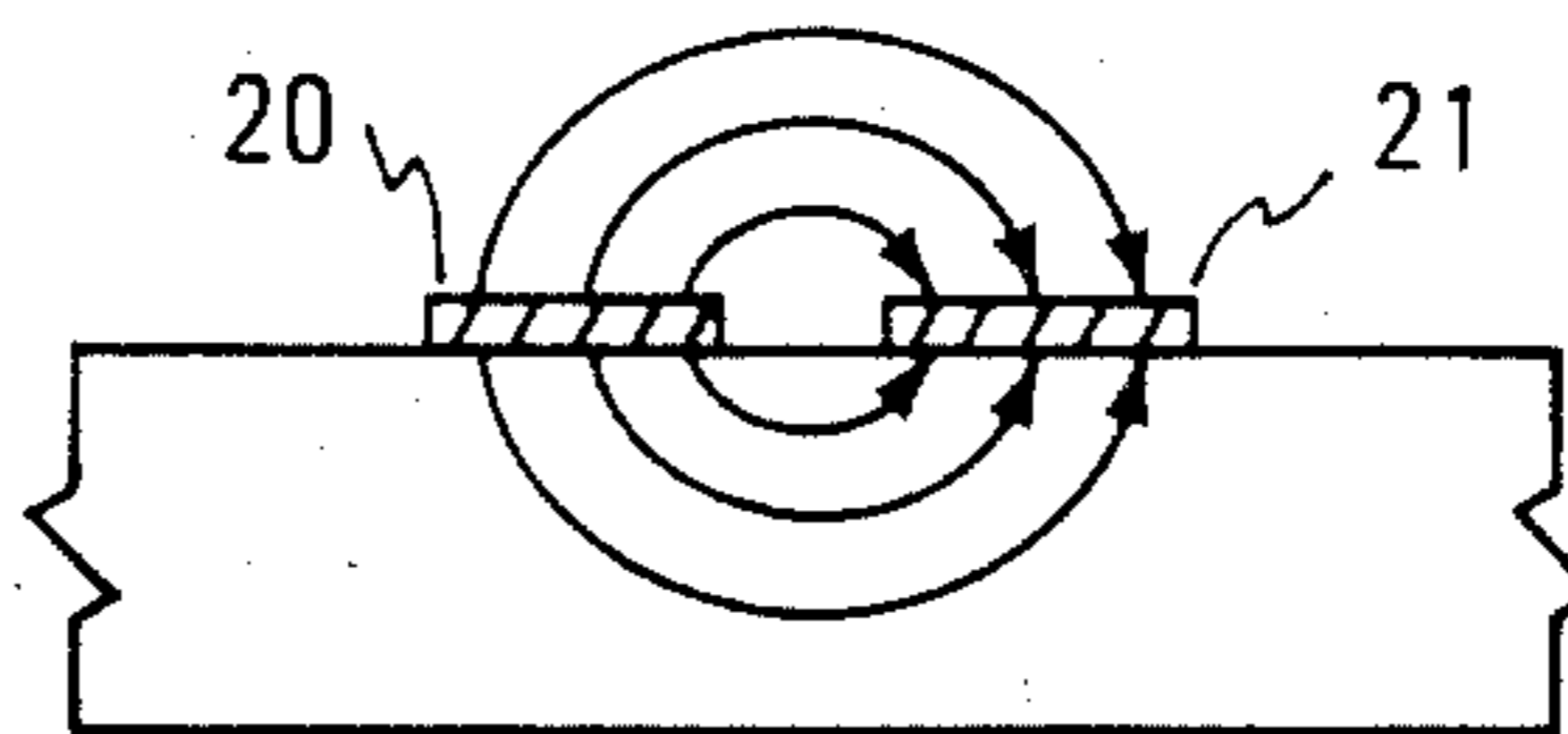
FIG. 3A COPLANAR STRIP
