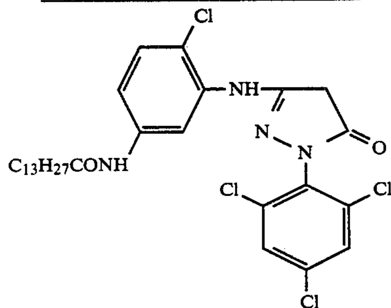
Comparative Magenta Coupler (D)
