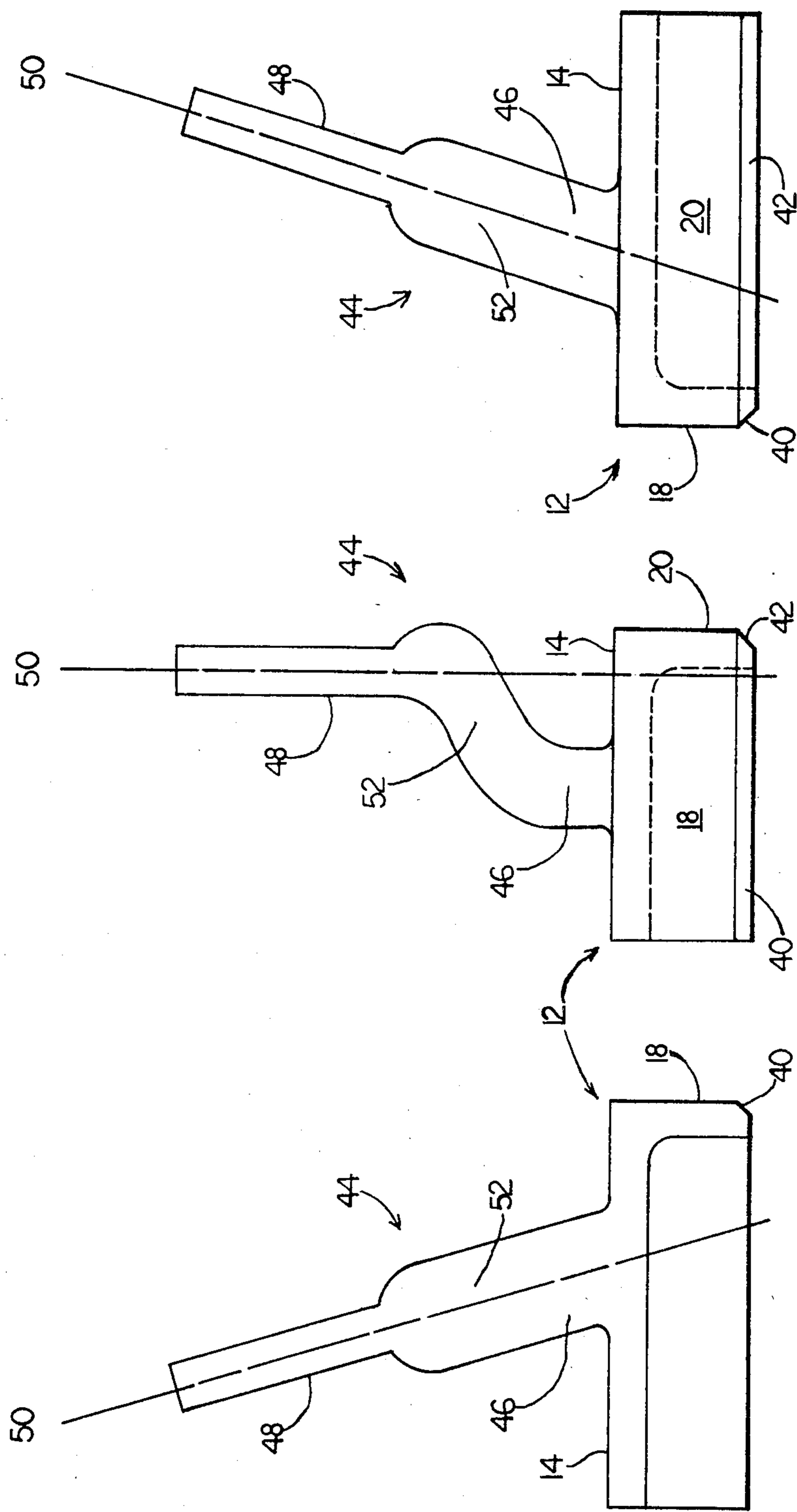
FIG. 2C
