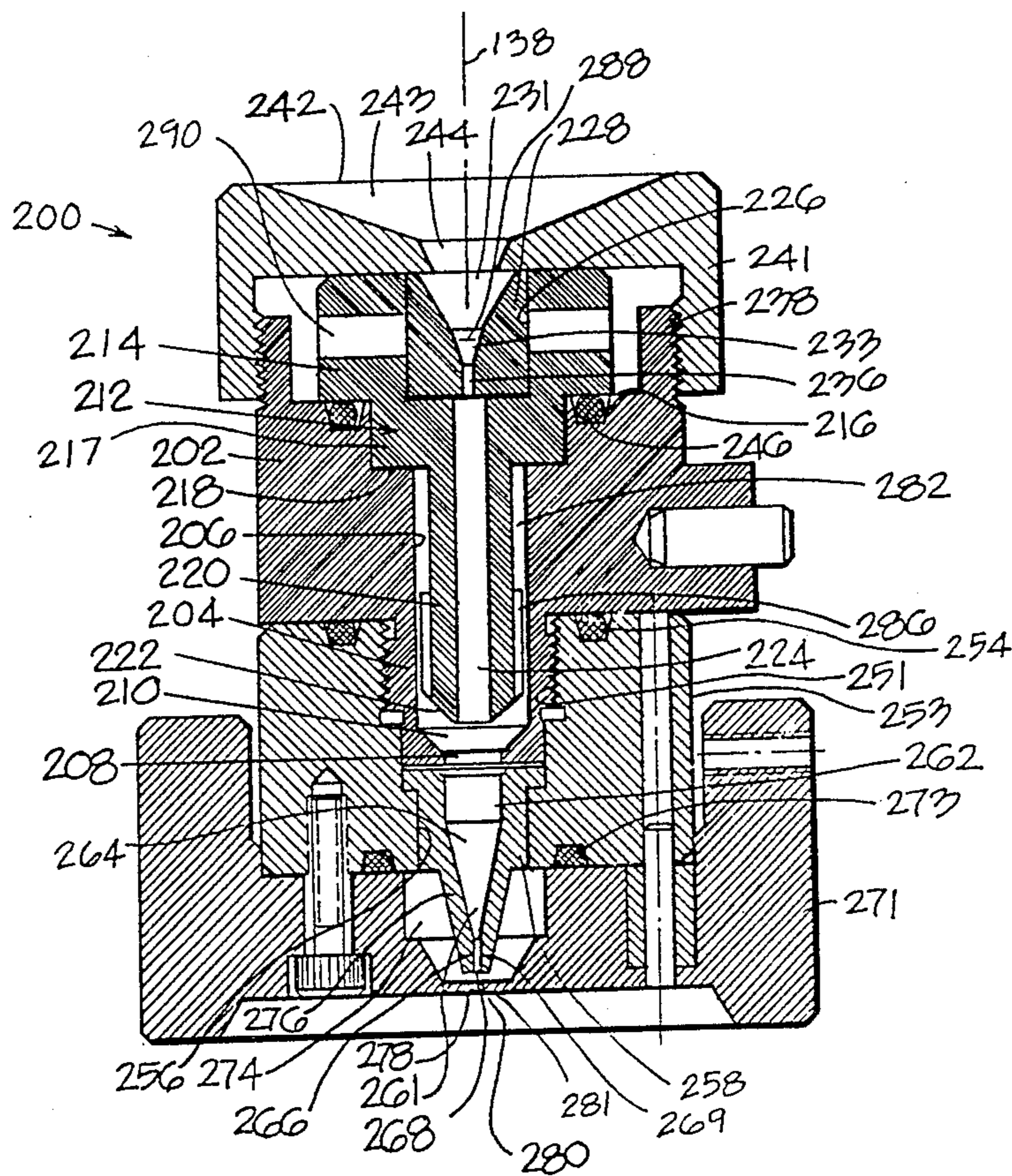
FIG. 6
