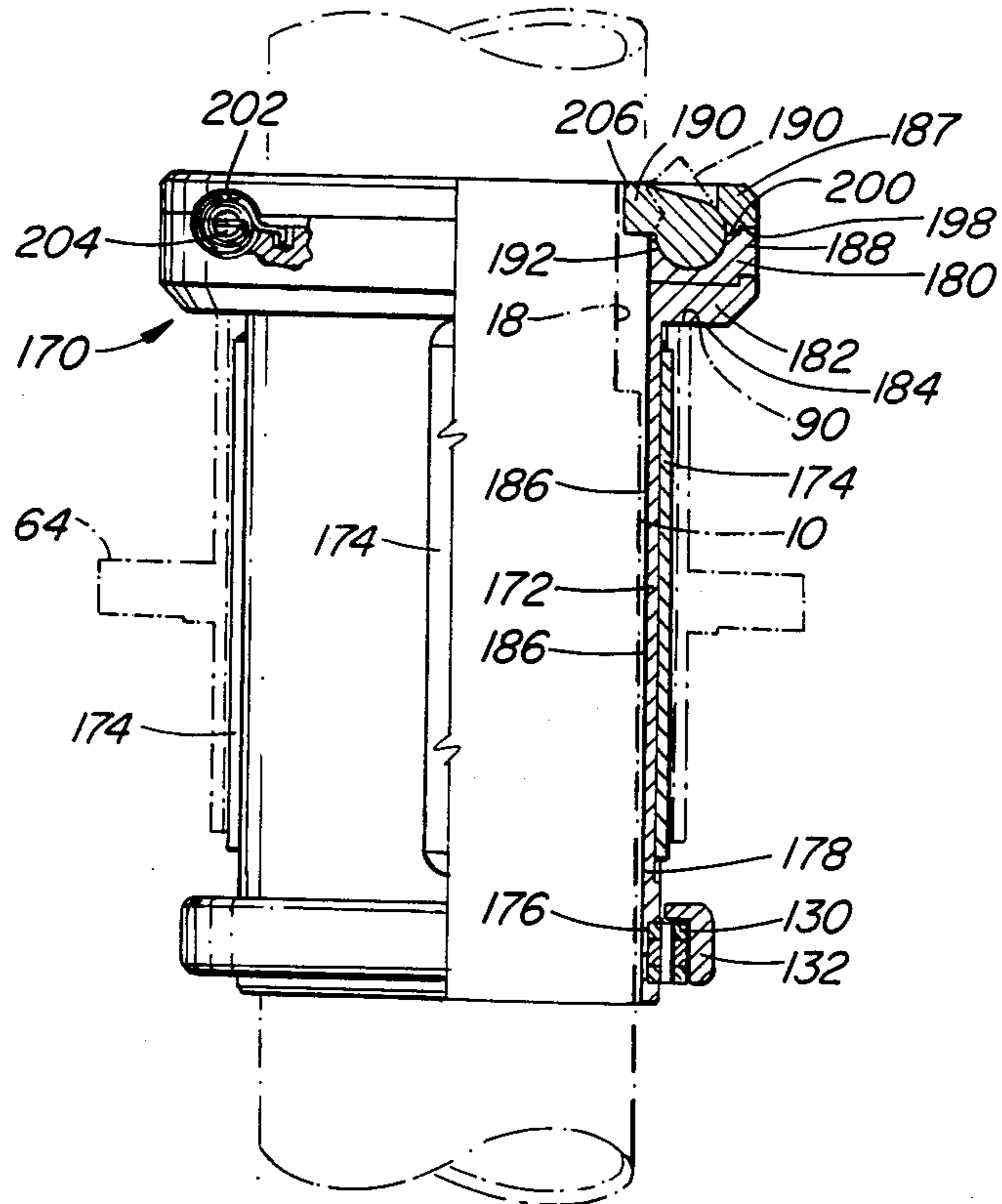
FIG. 8
