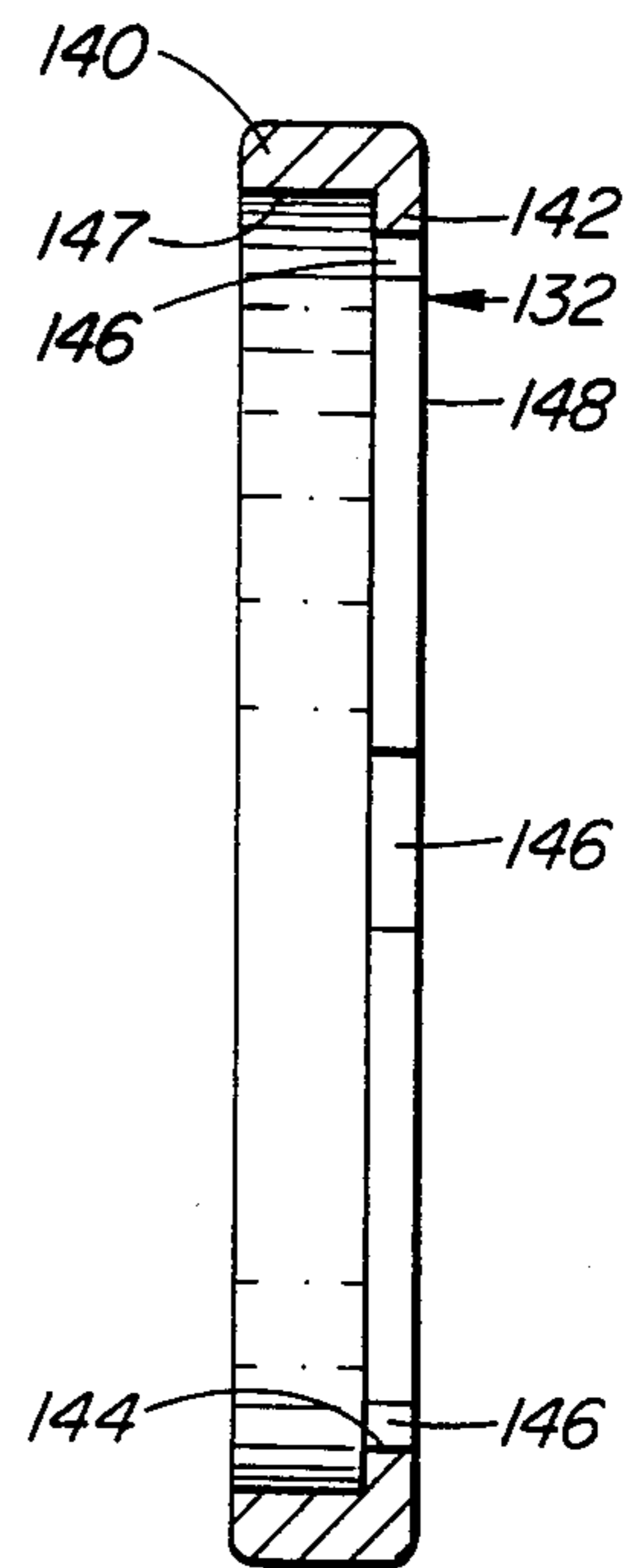
FIG. 15
