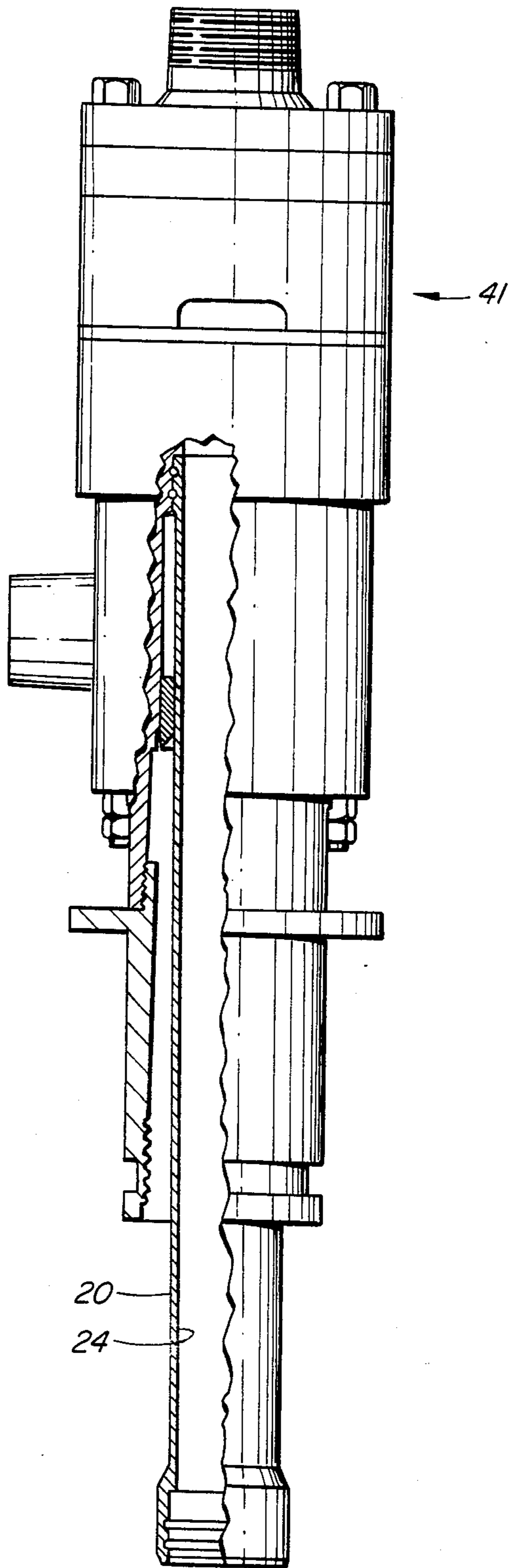
FIG. 5a
