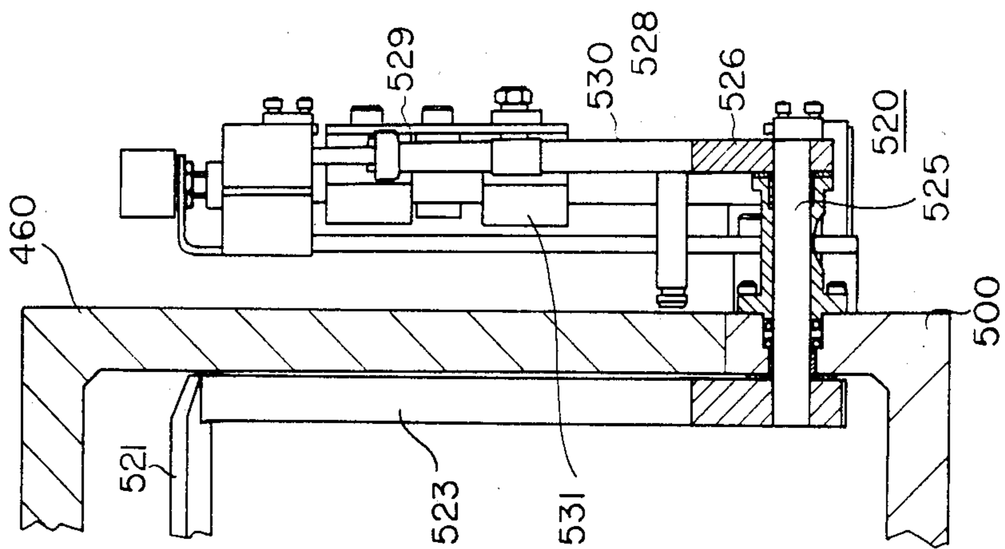
FIG. 60
