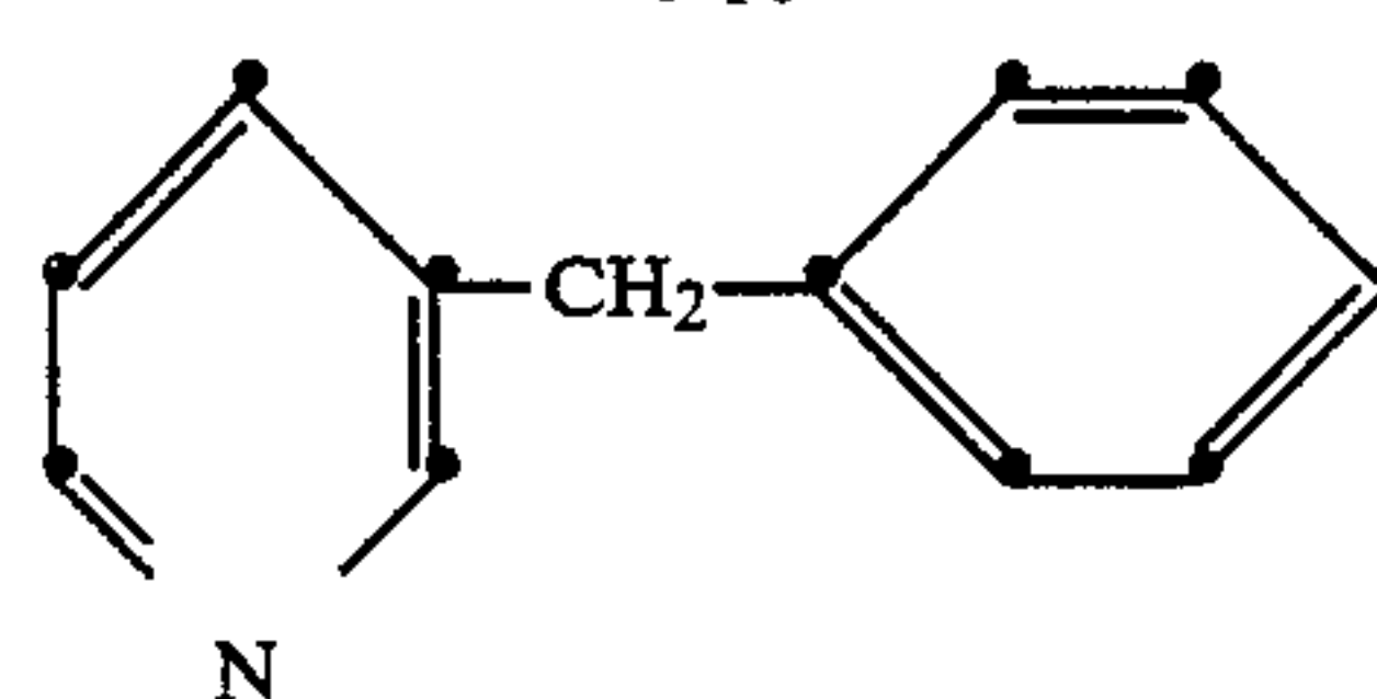
3-Benzylpyridine:
