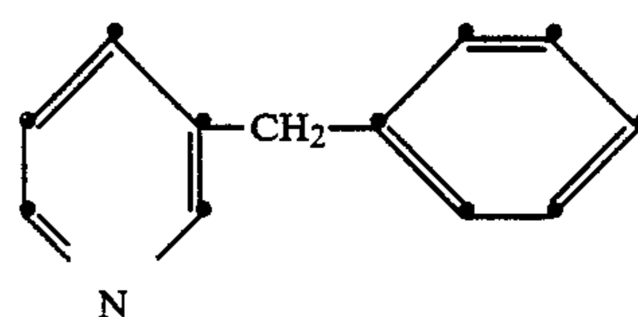
3-Benzylpyridine:
