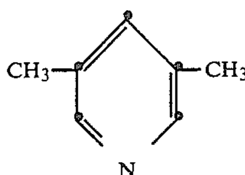
3,5-Lutidine:
