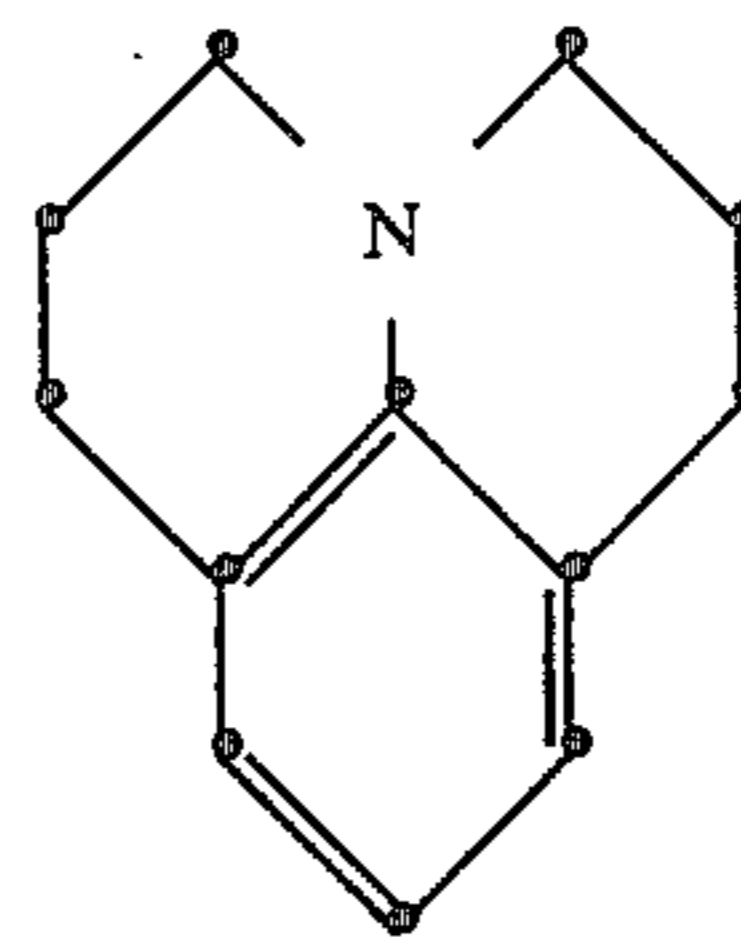
julolidine AN-2
