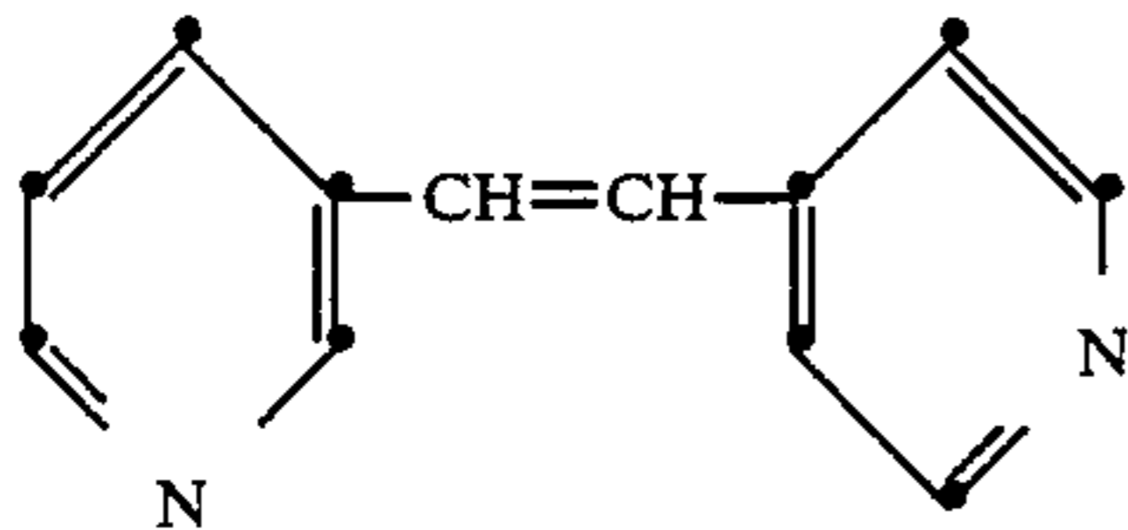
Trans-1-(3-pyridyl)-2-(4-pyridyl)ethylene:
