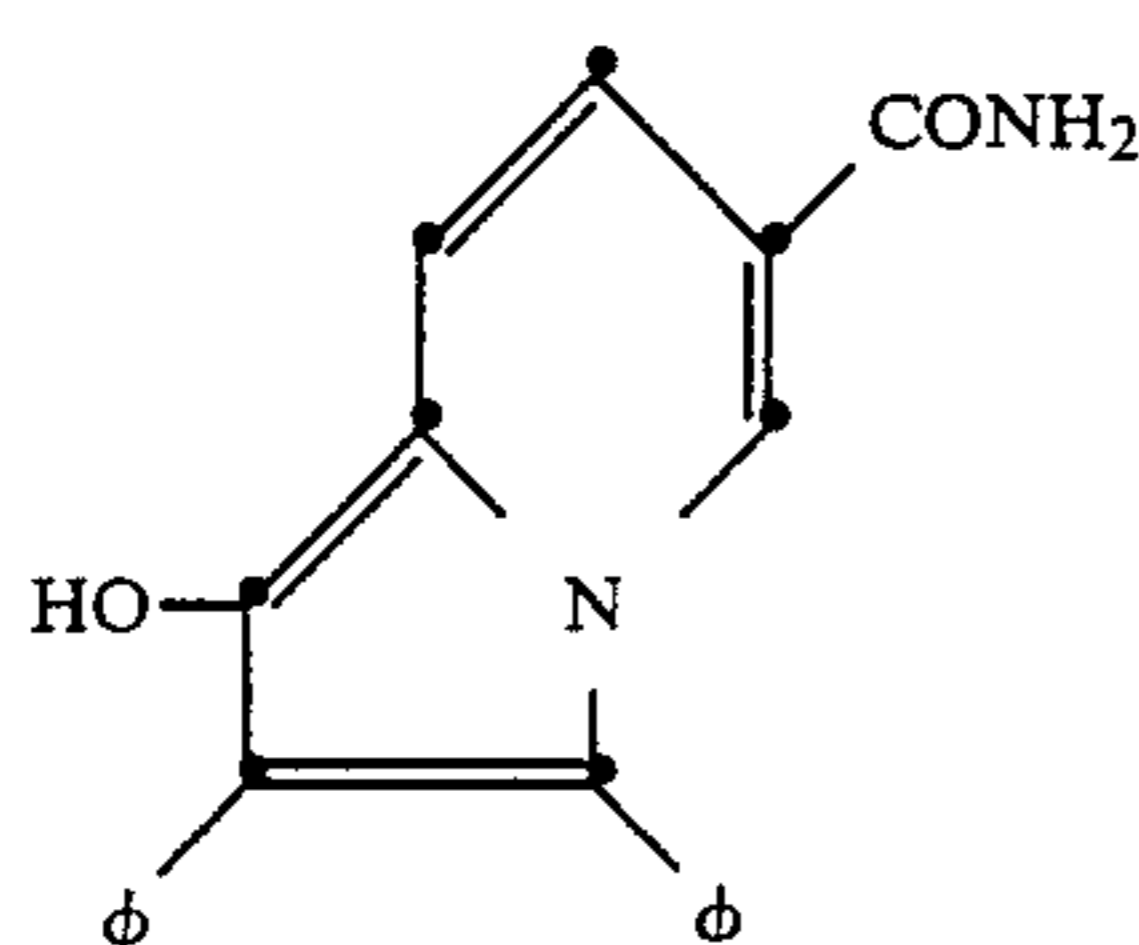
8-carboethoxy-2,3-diphenyl-1-indolizinol
