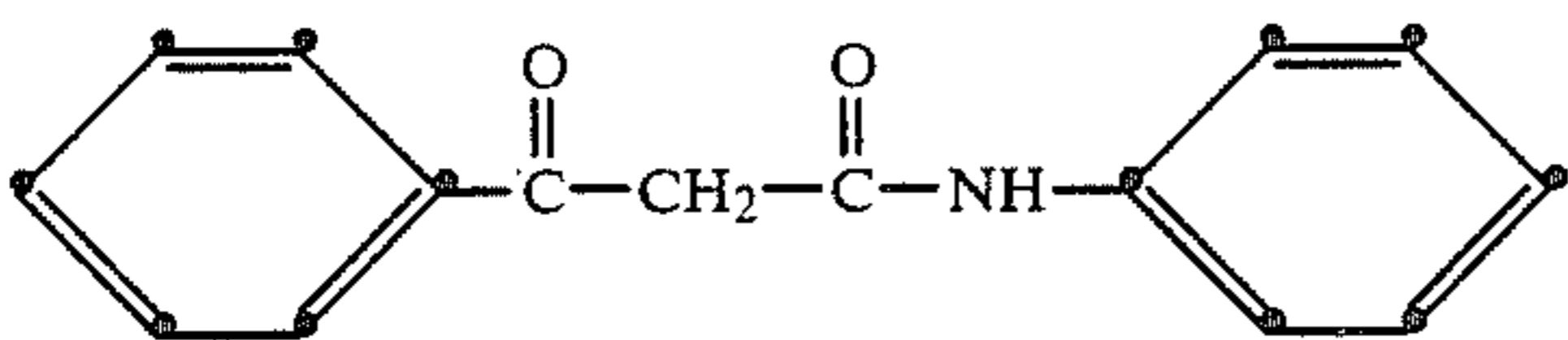
1-anilino-3-phenyl-1,3-propanedione
