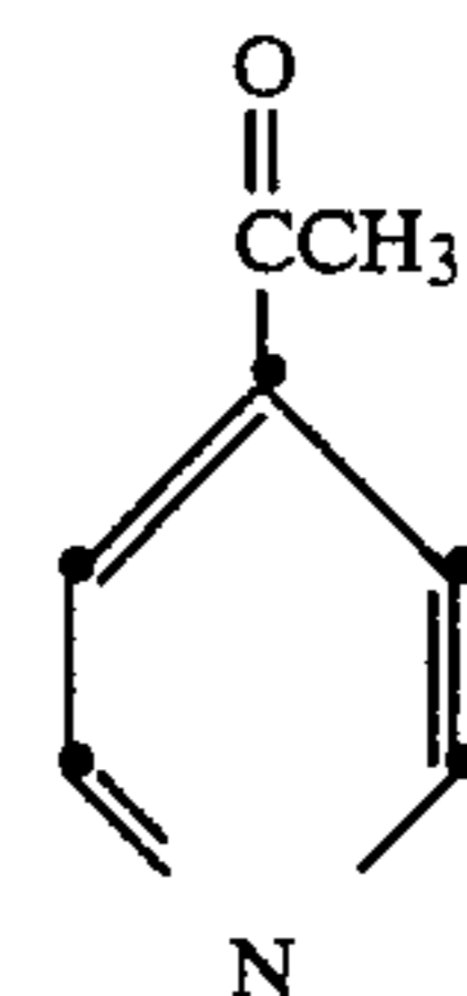
4-Acetylpyridine:
