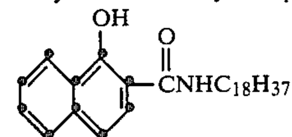
2-octadecyl aminocarbonyl-1-naphthol
