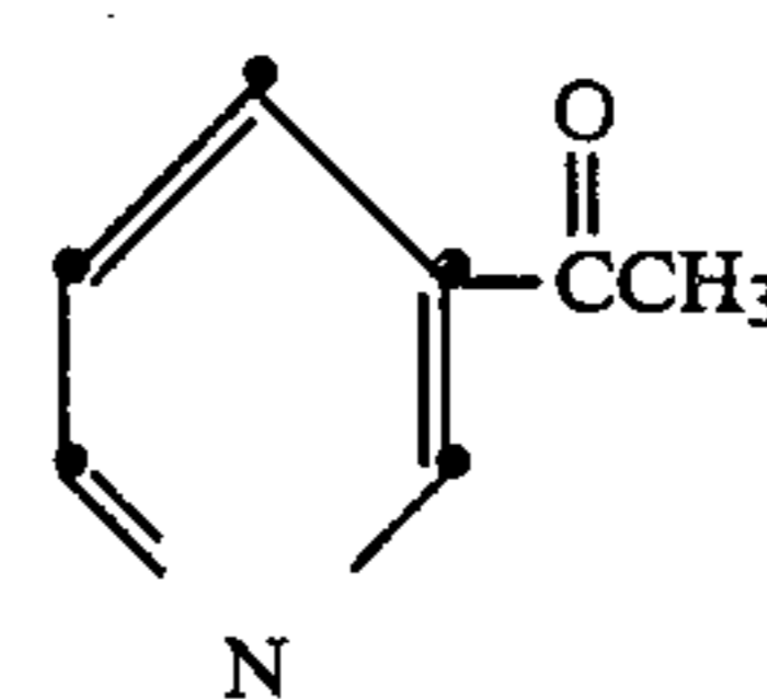
3-Acetylpyridine:
