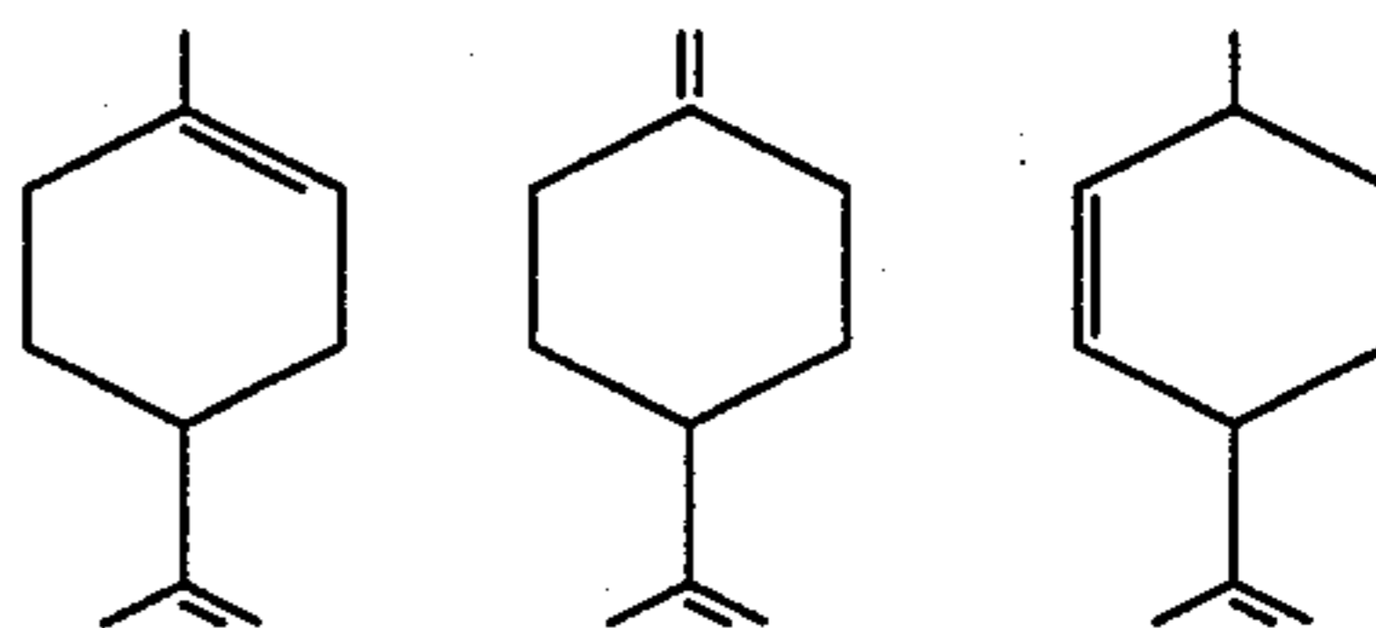
Dipentene (Limonene) 1,8-p- Menthadiene Trans-iso- Limonene
