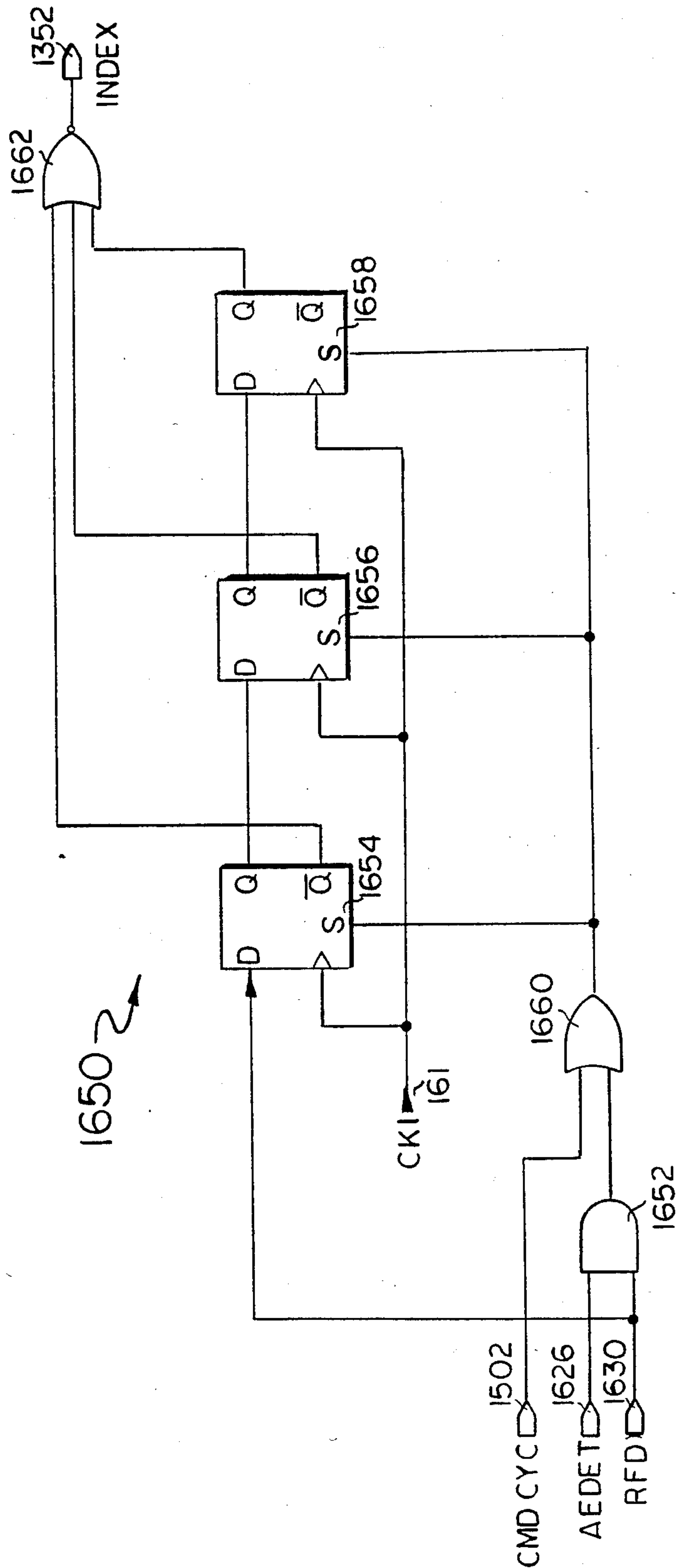
FIG. 29
