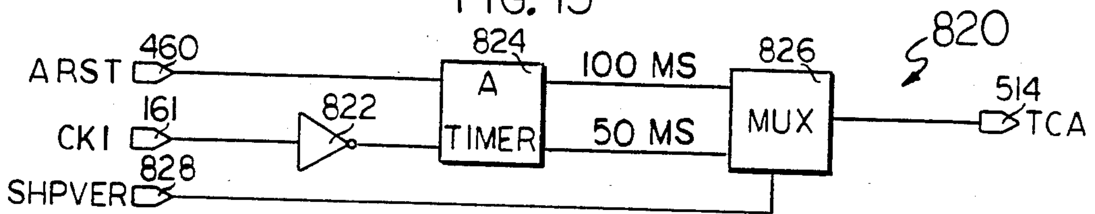
FIG. 16
