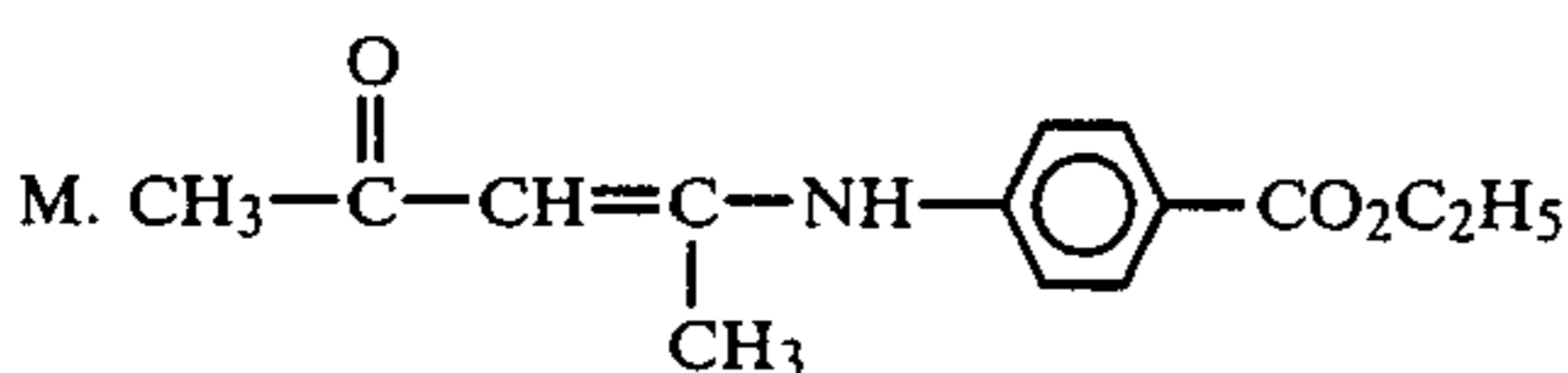
4-(p-carboxyethylphenyl)-amino-3-pentene-2-one
