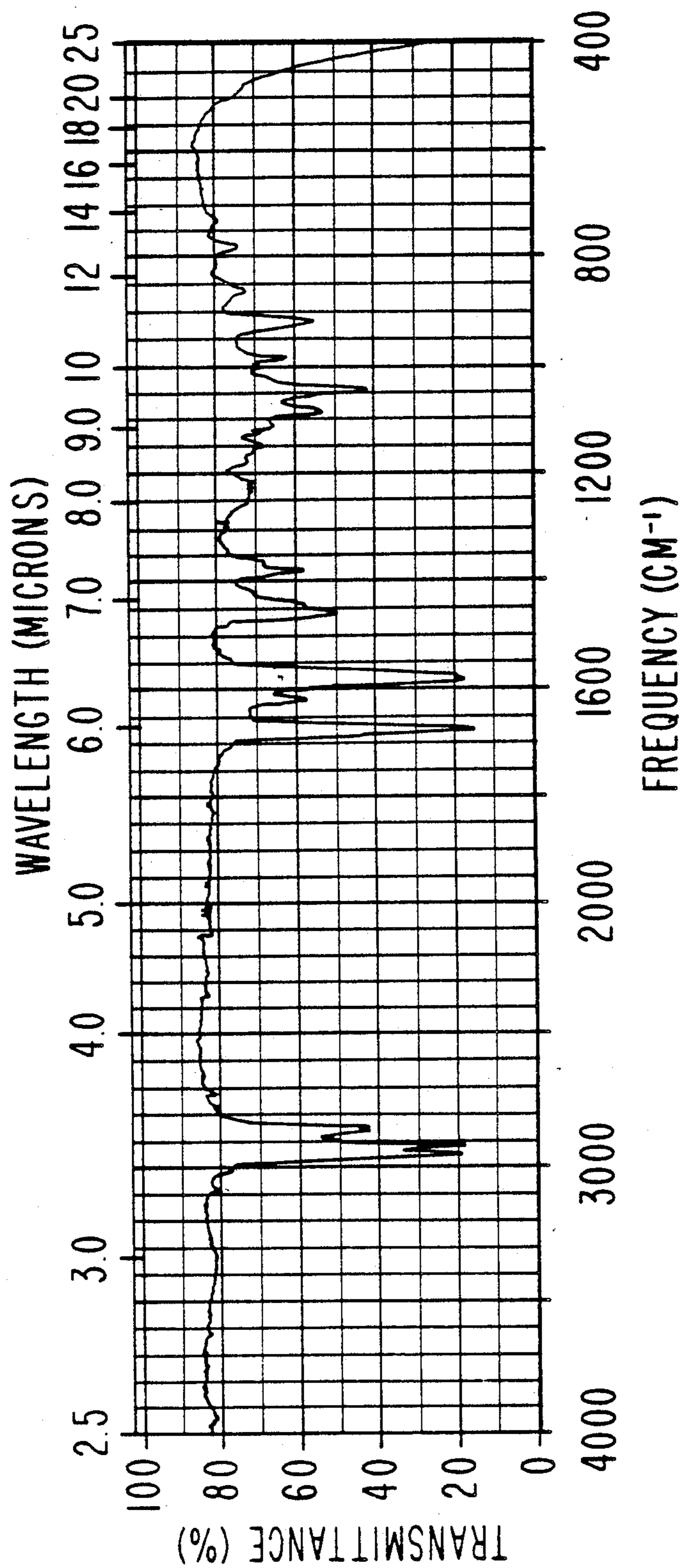
IR SPECTRUM FOR EXAMPLE VII B.
