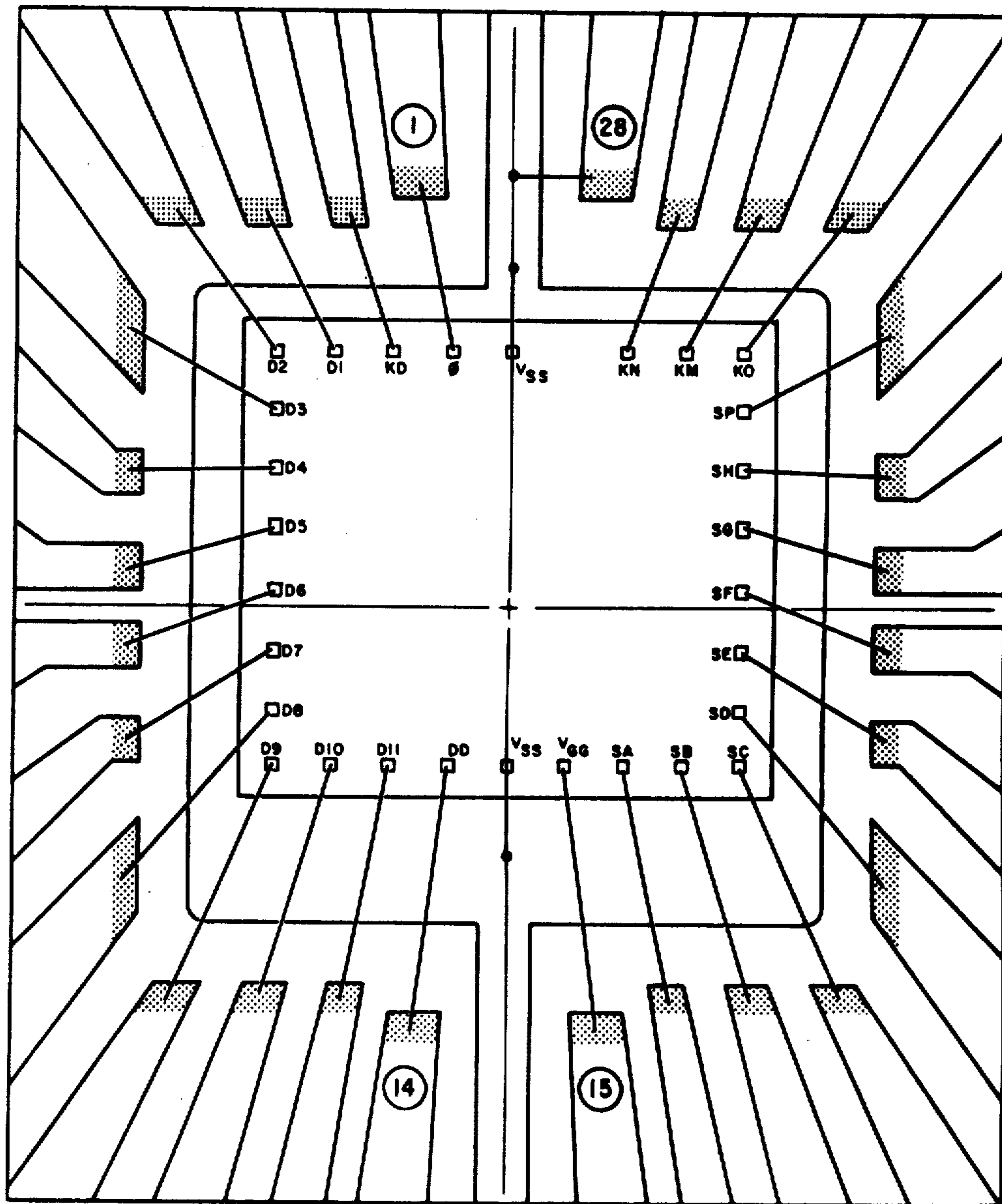
Fig. 17
