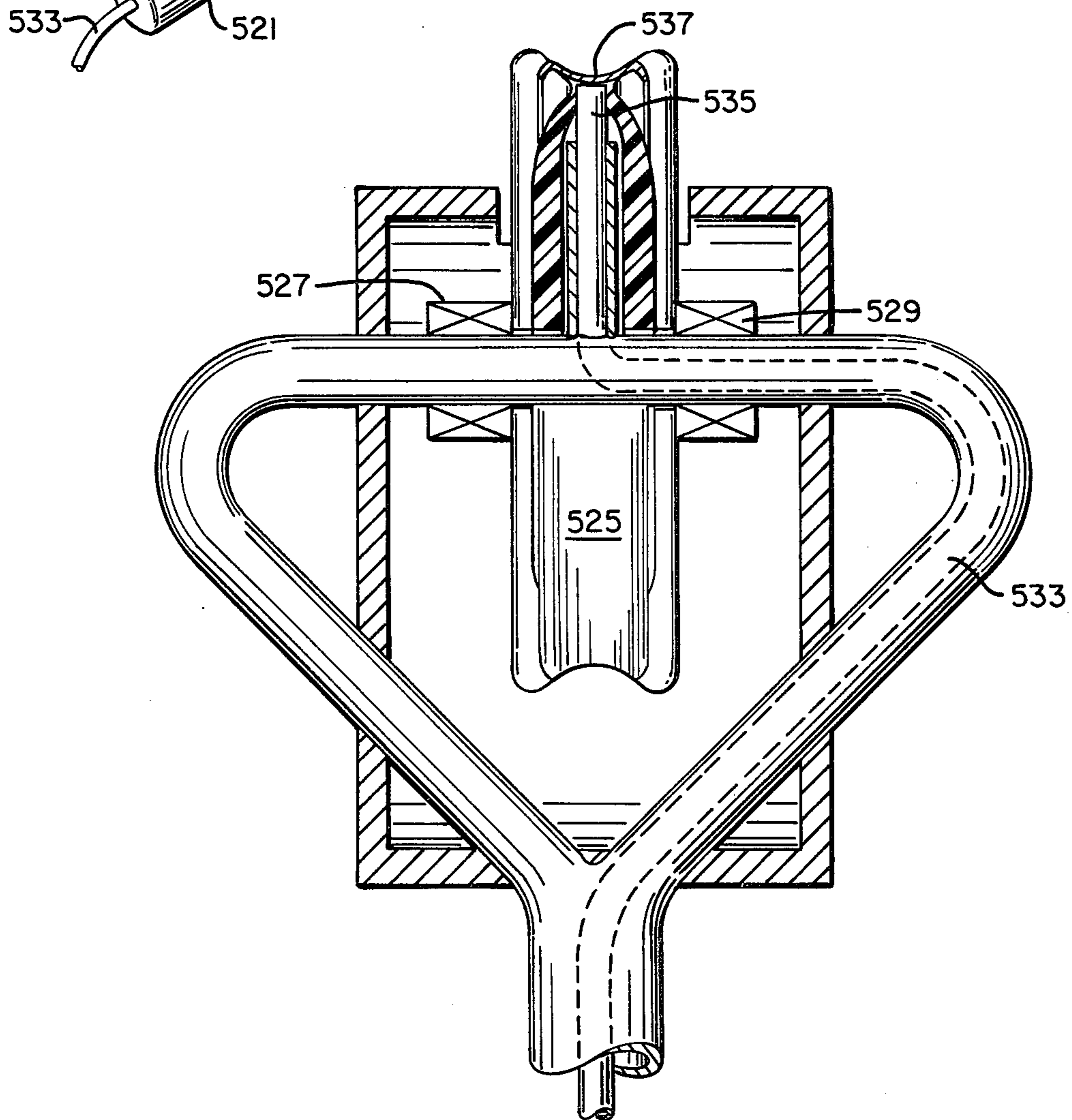
FIG. 22A
