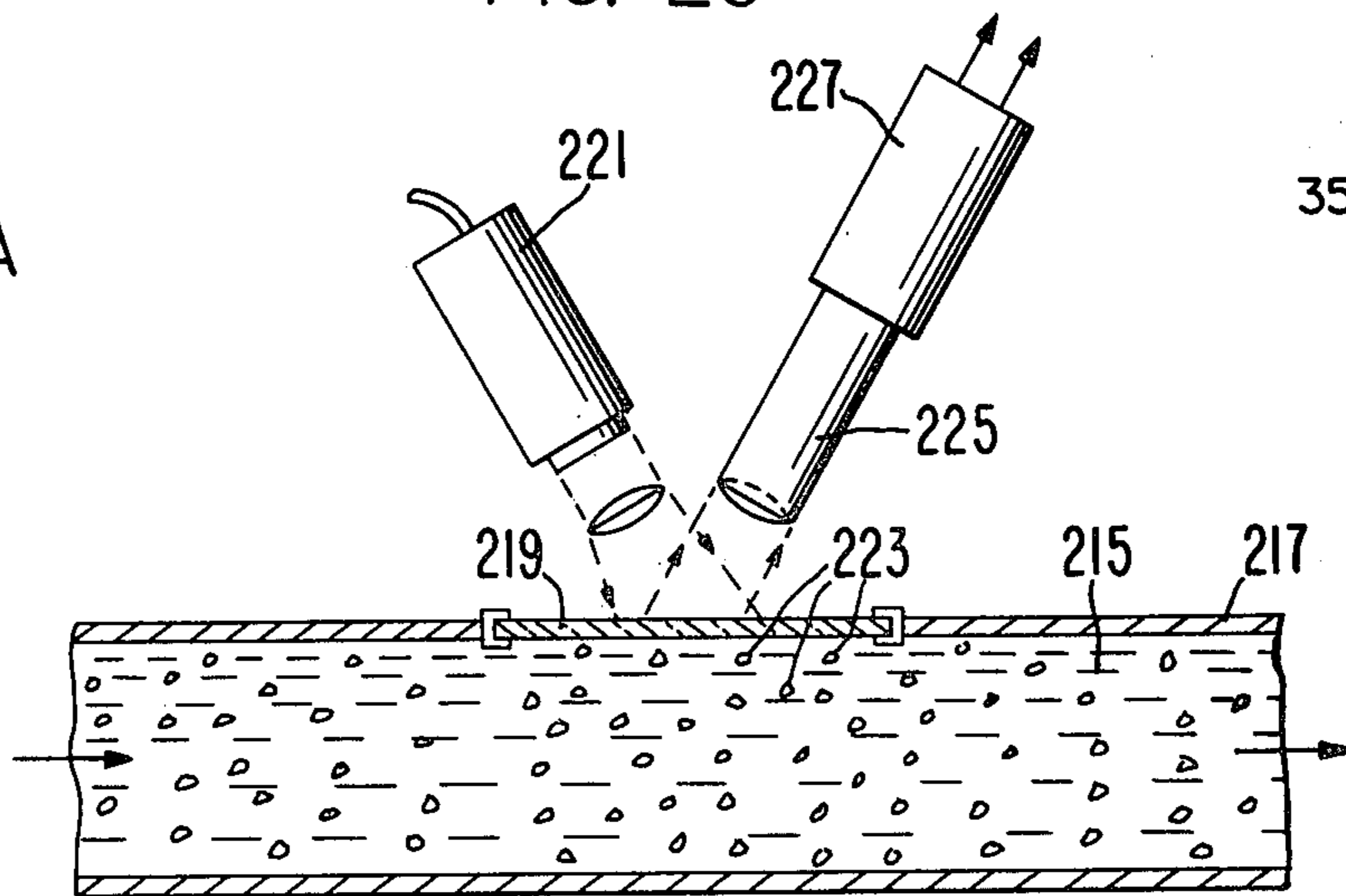
FIG. 13
