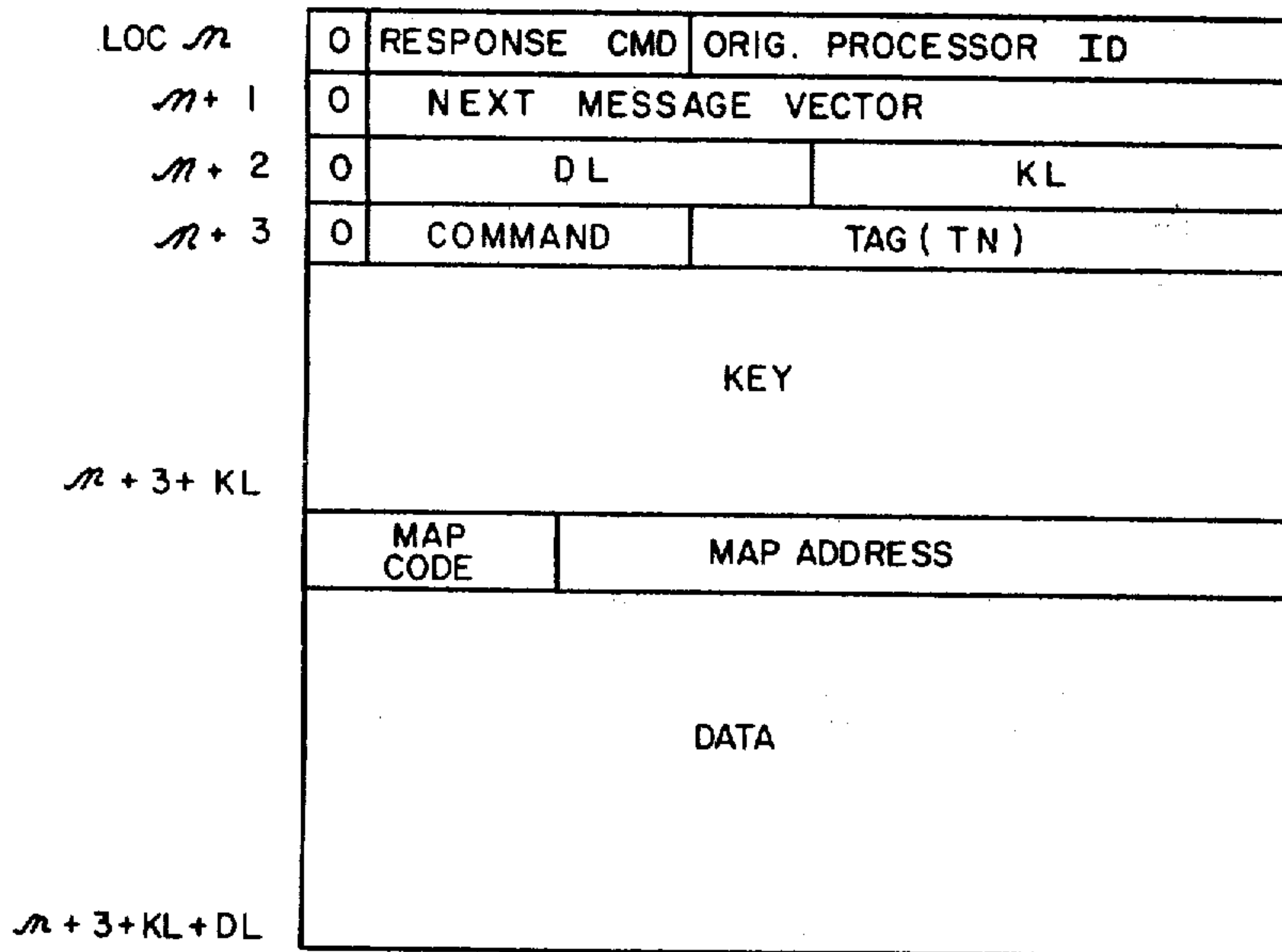
A. SEND MESSAGE FORMAT
