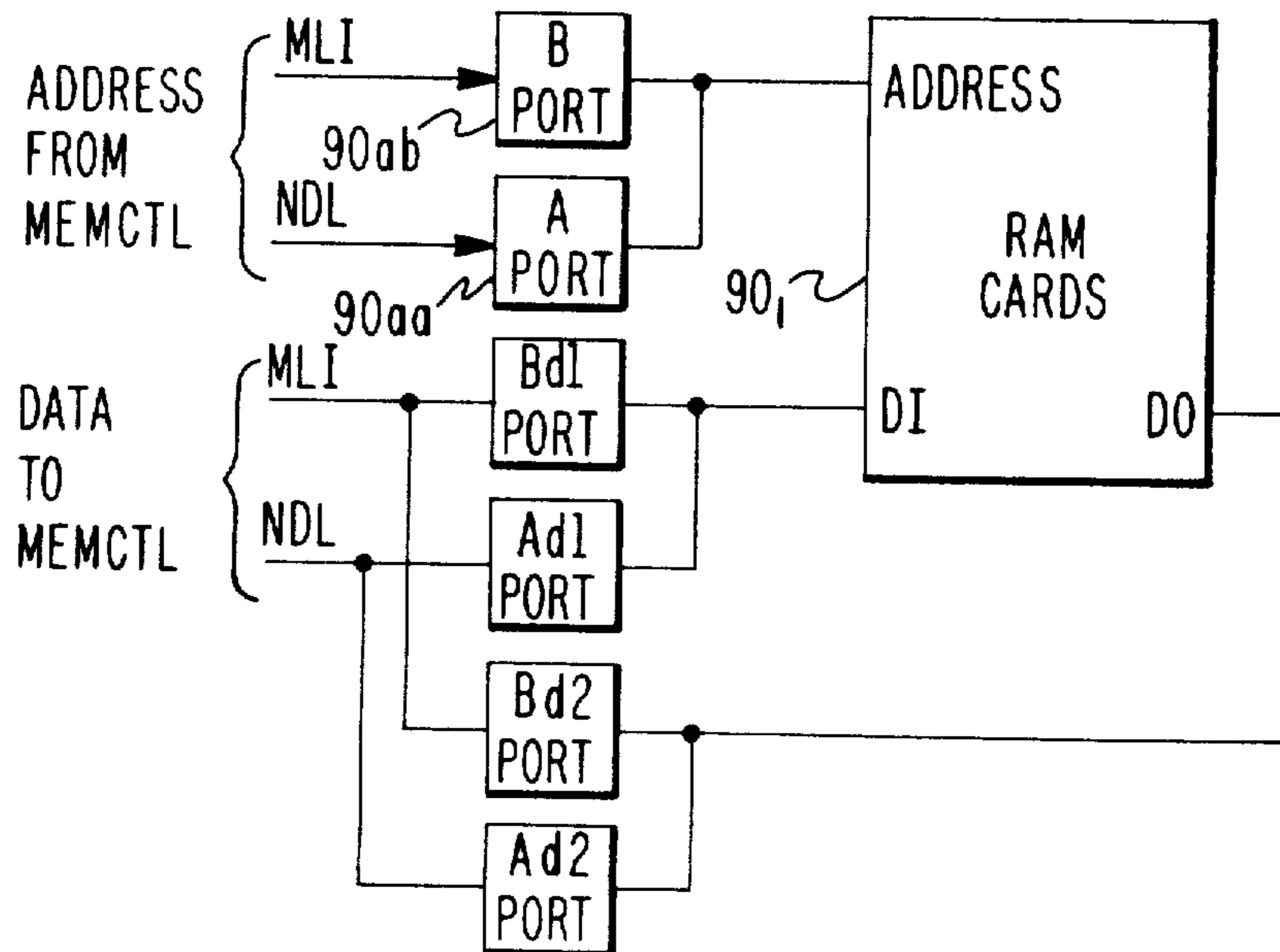
FIG. 12. 32 KB RAM BLOCK DIAGRAM.
