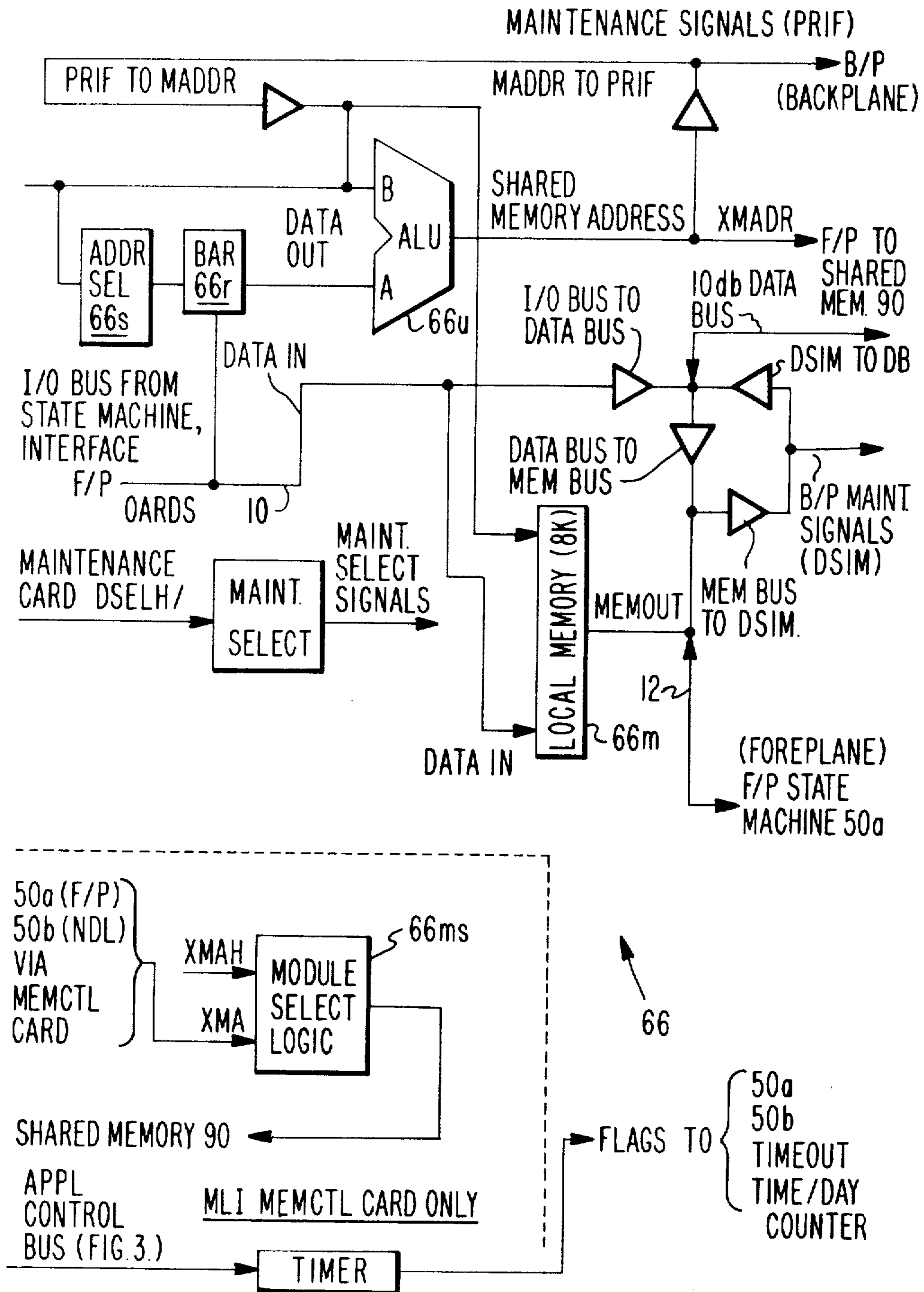
FIG. 11. MEMCTL BLOCK DIAGRAM.
