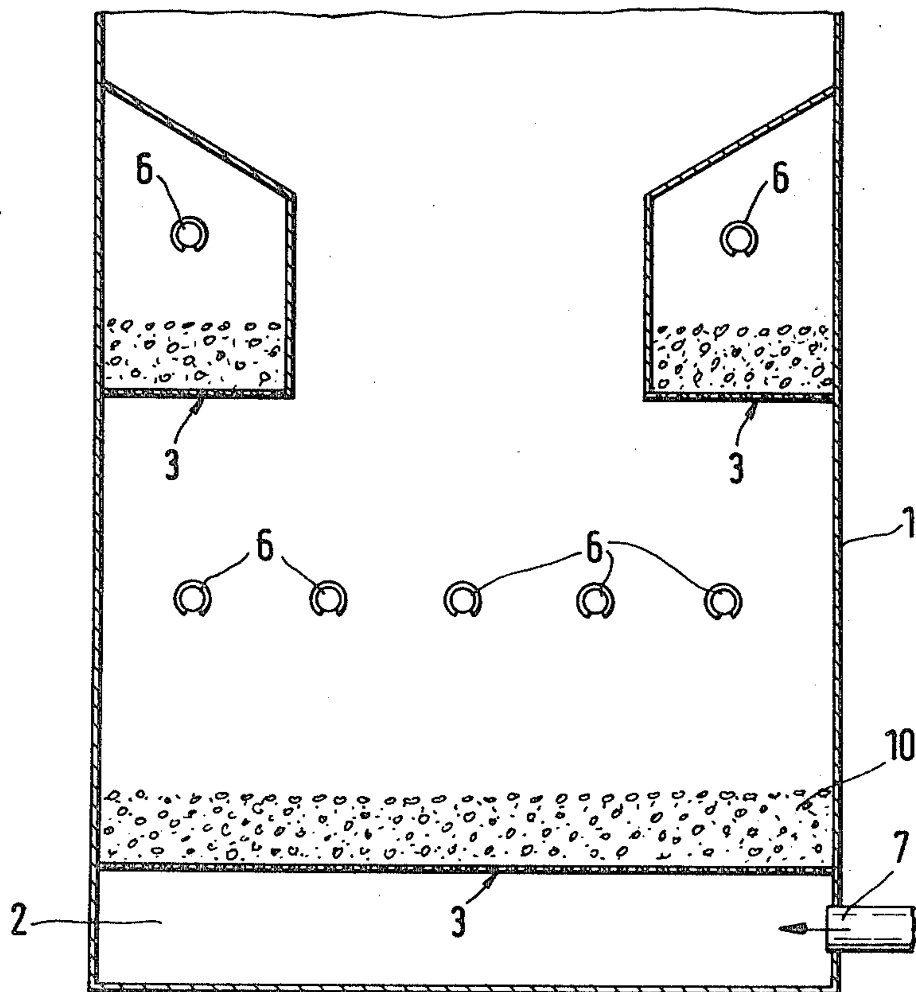
FIG. 5
