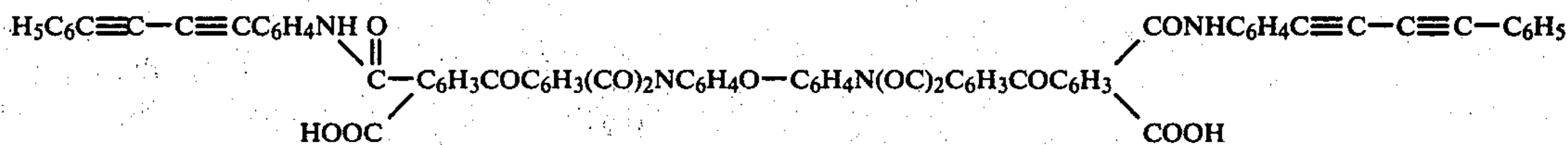
(Amic-Acid #1)
