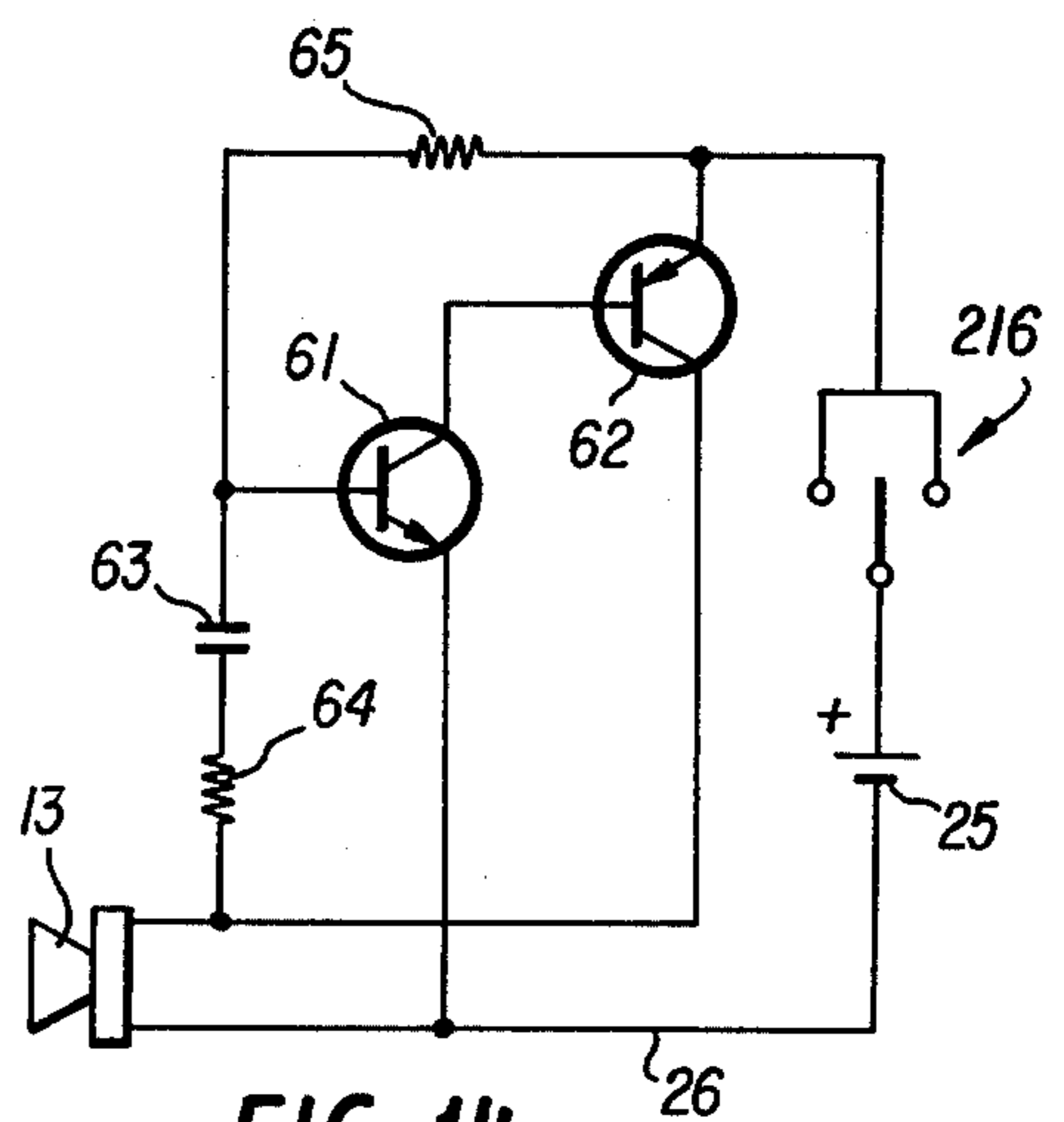
FIG. 14
