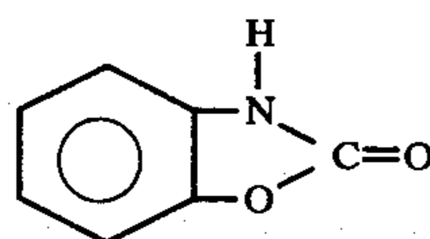
2-Benzoxazdinone
