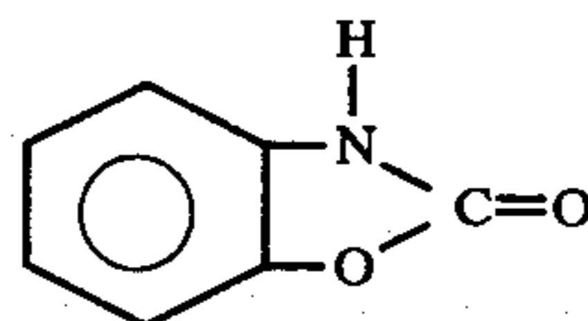
2-Benzoxazdinone
