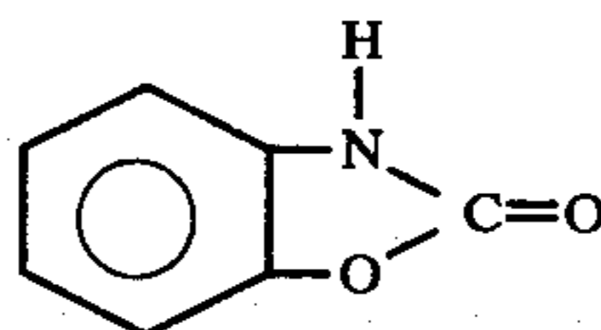
2-Benzoxazdinone
