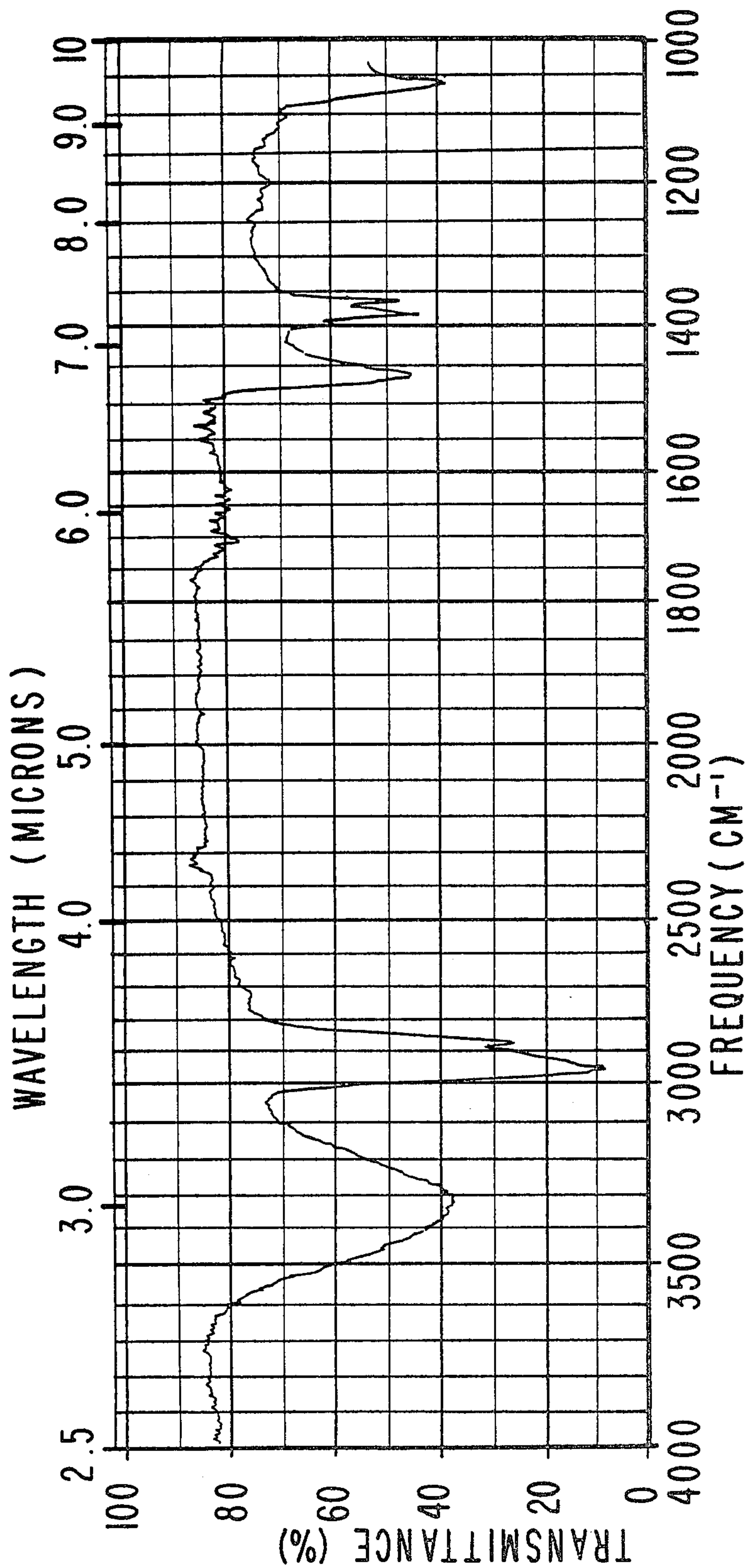
IR SPECTRUM FOR EXAMPLE II, DIISOUNDECANOL.
