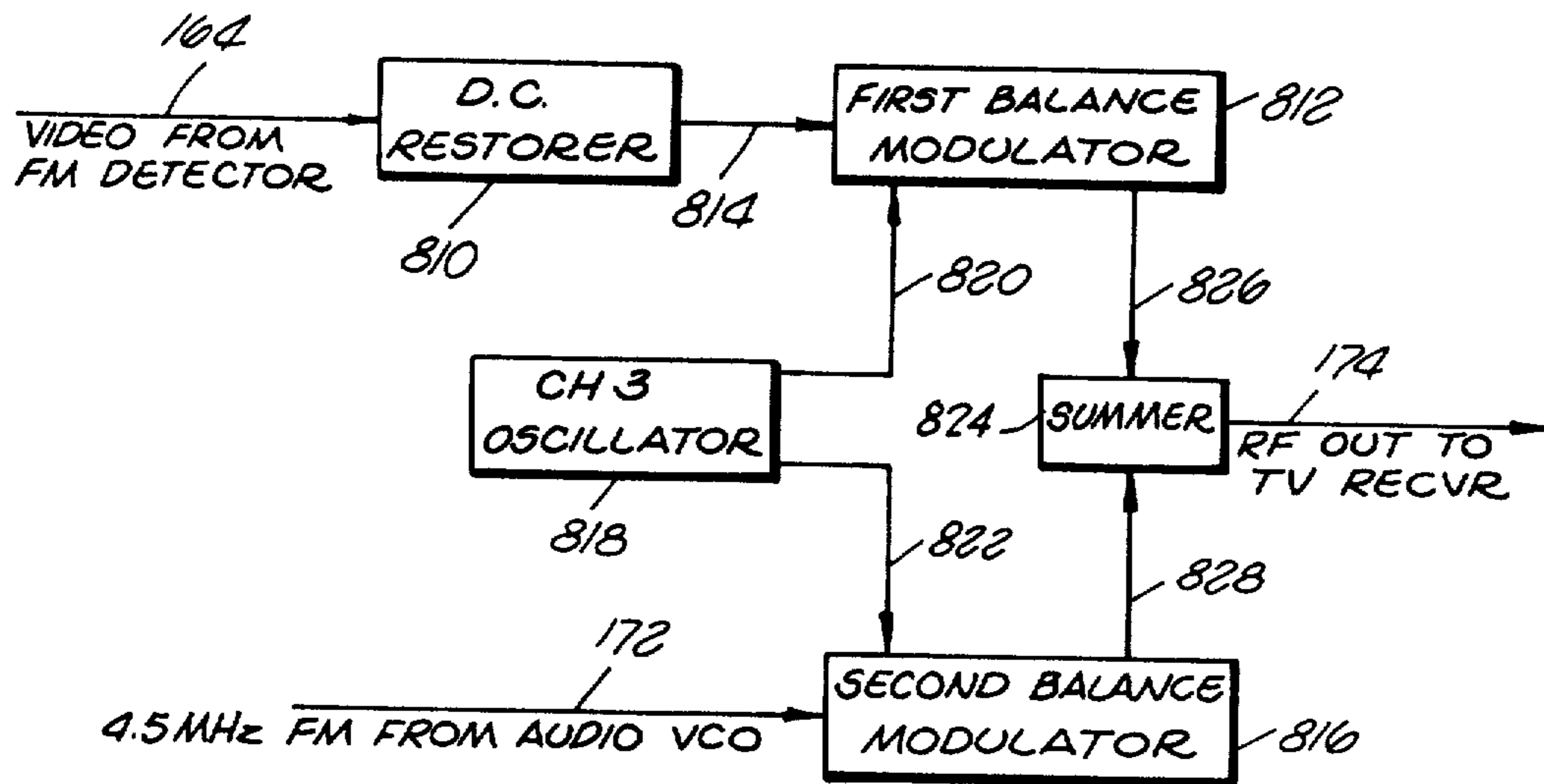
FIG. 24 RF MODULATOR
