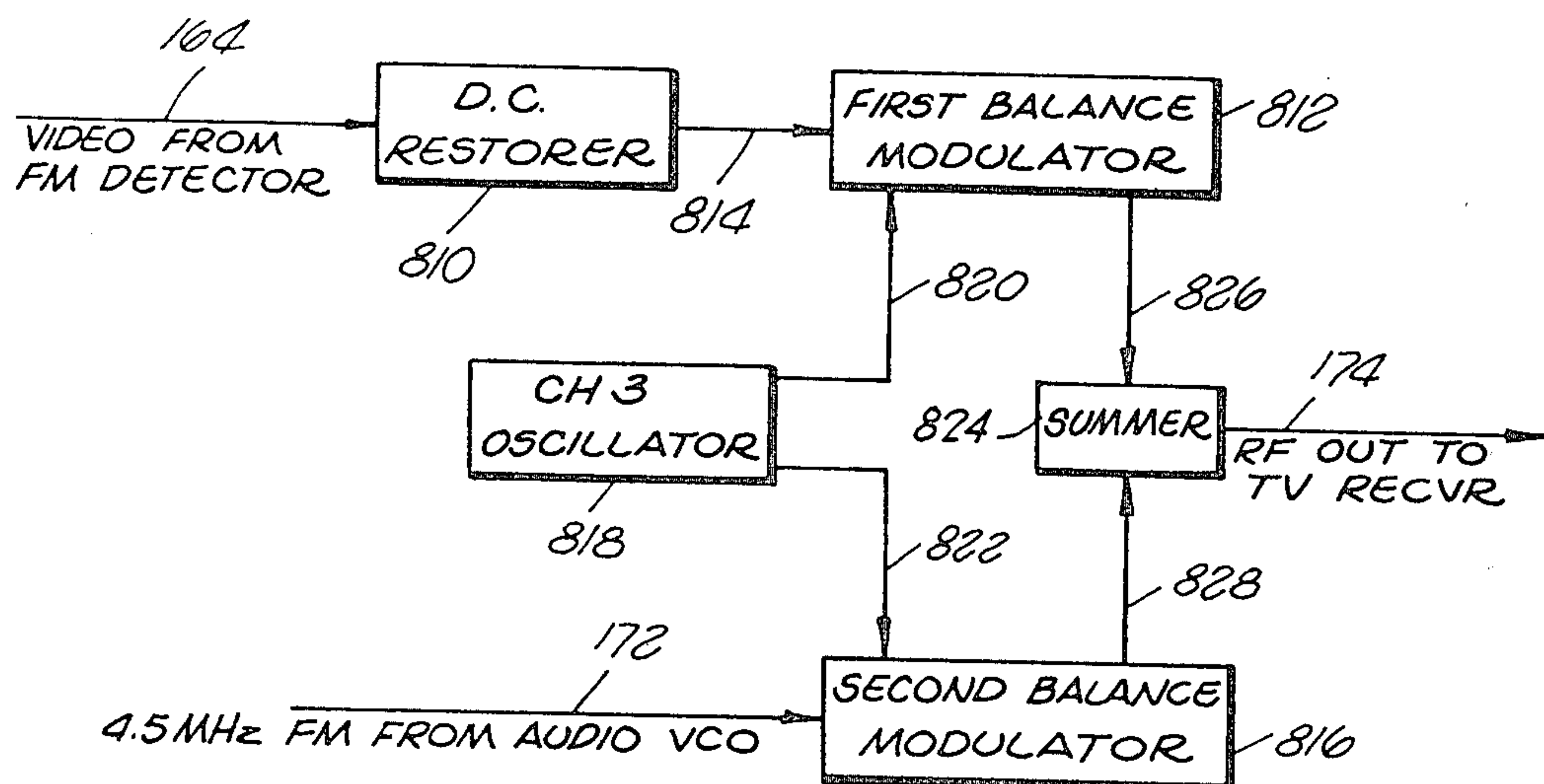
FIG. 24 RF MODULATOR
