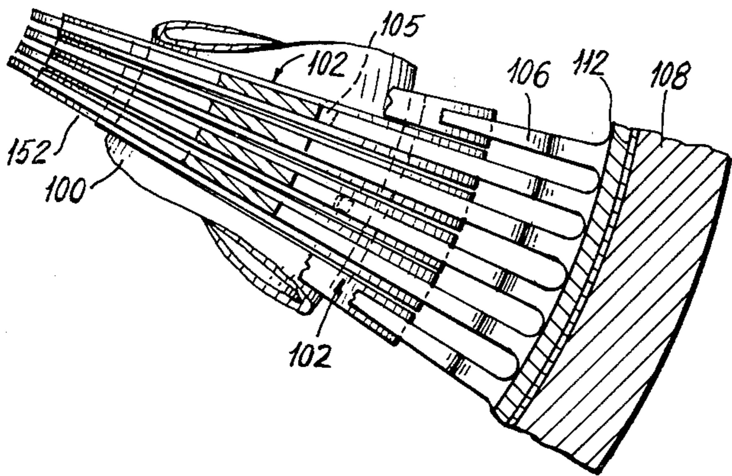
Fig. 7A.
