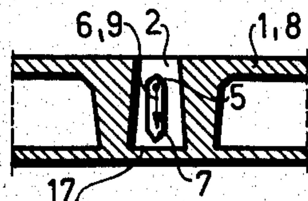
Fig. 12 K-K
