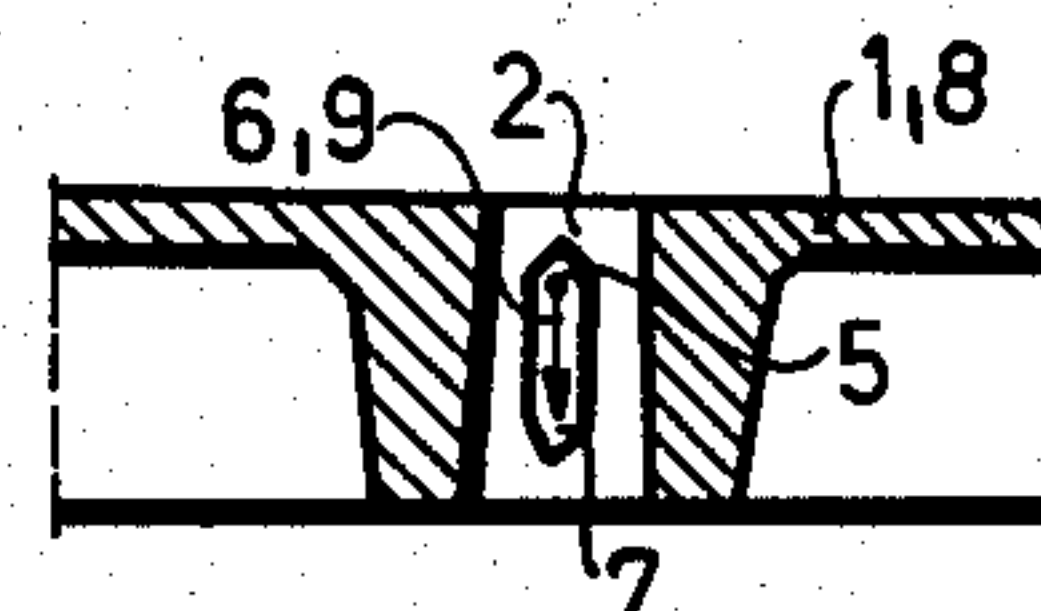
Fig. 9 G-G
