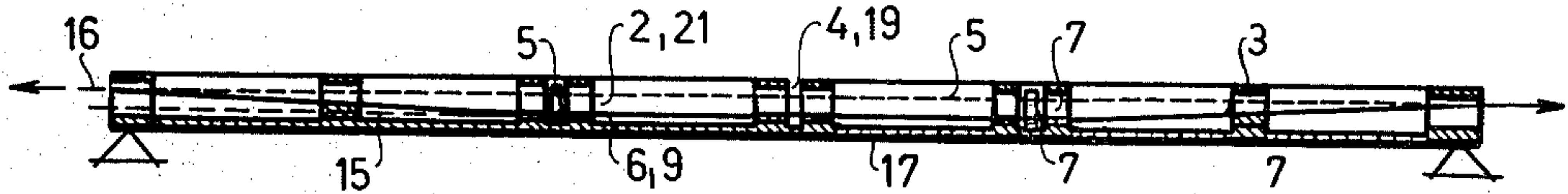
Fig. 15 H-H
