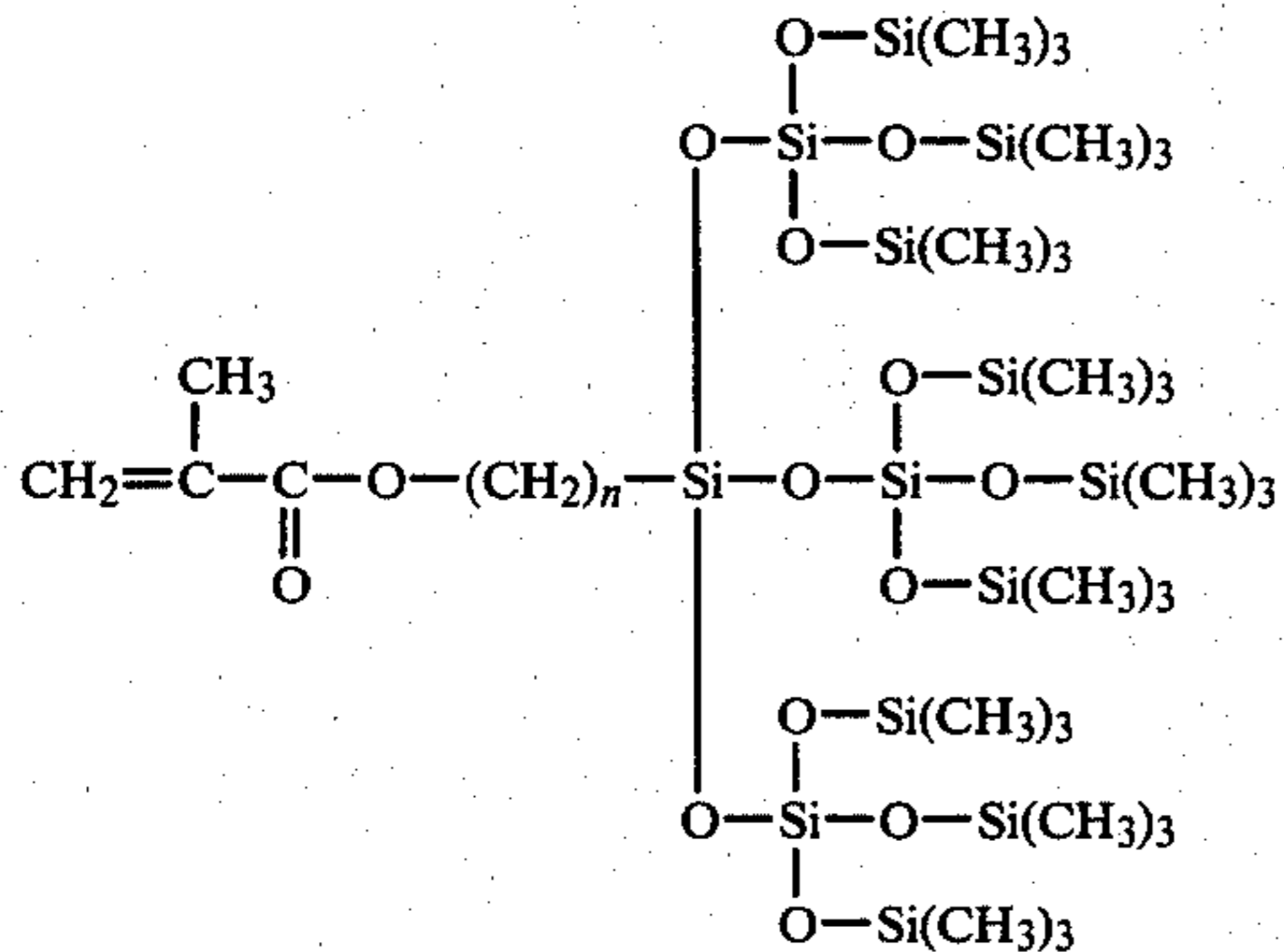
tris(tris-trimethylsiloxy-siloxanyl)methacryloxyalkylsilane
