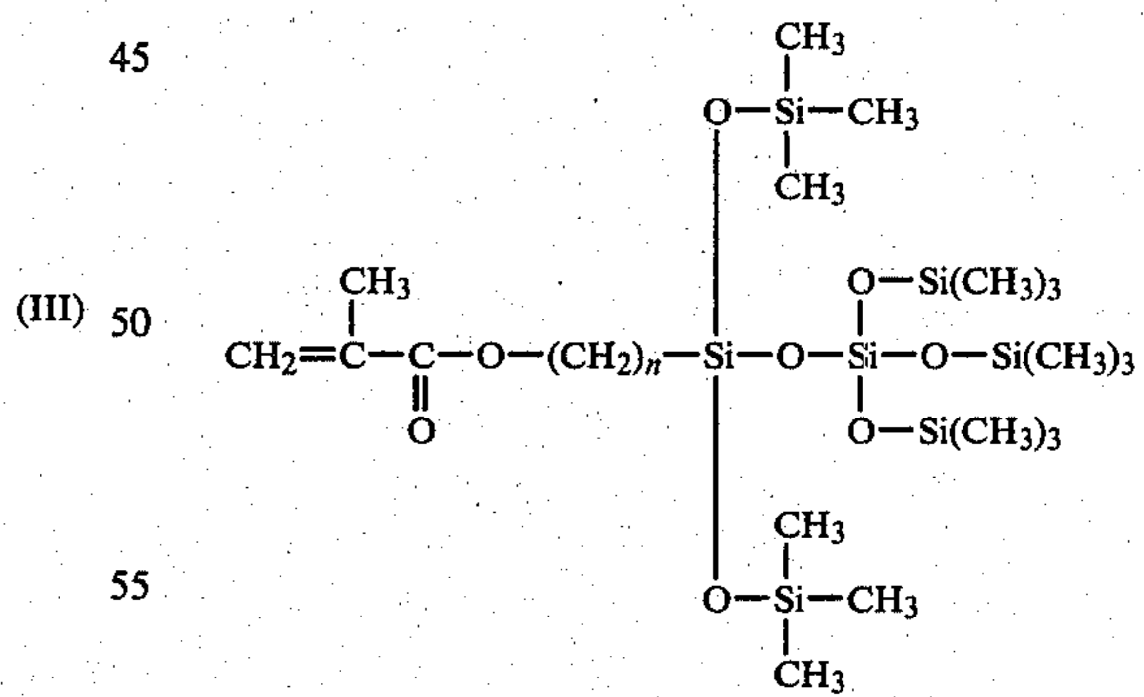
mono(tris-trimethylsiloxy-siloxanyl)bis(trimethylsiloxy) methacryloxyalkylsilane
