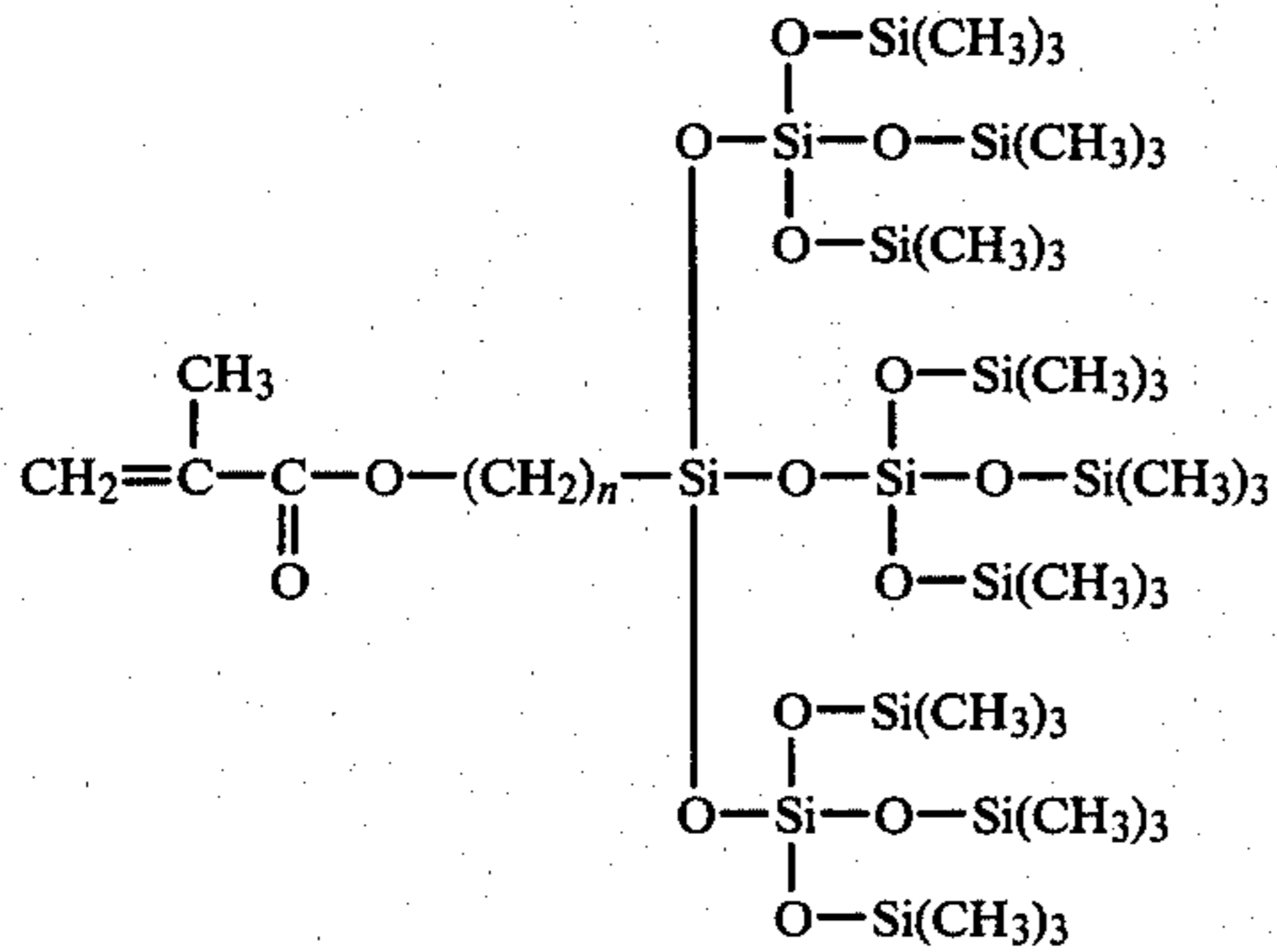
tris(tris-trimethylsiloxy-siloxanyl)methacryloxyalkylsilane
