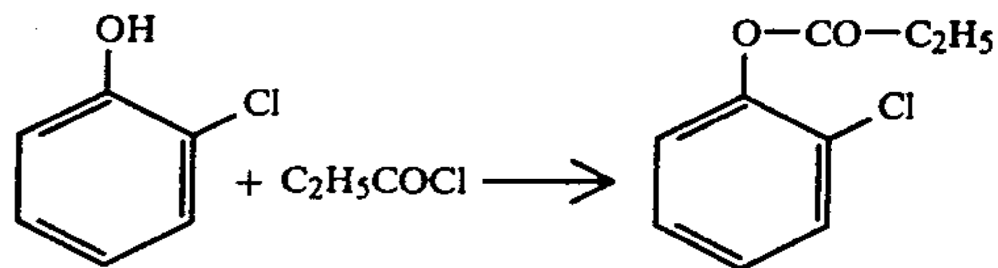
A. o -Chlorophenyl propionate
