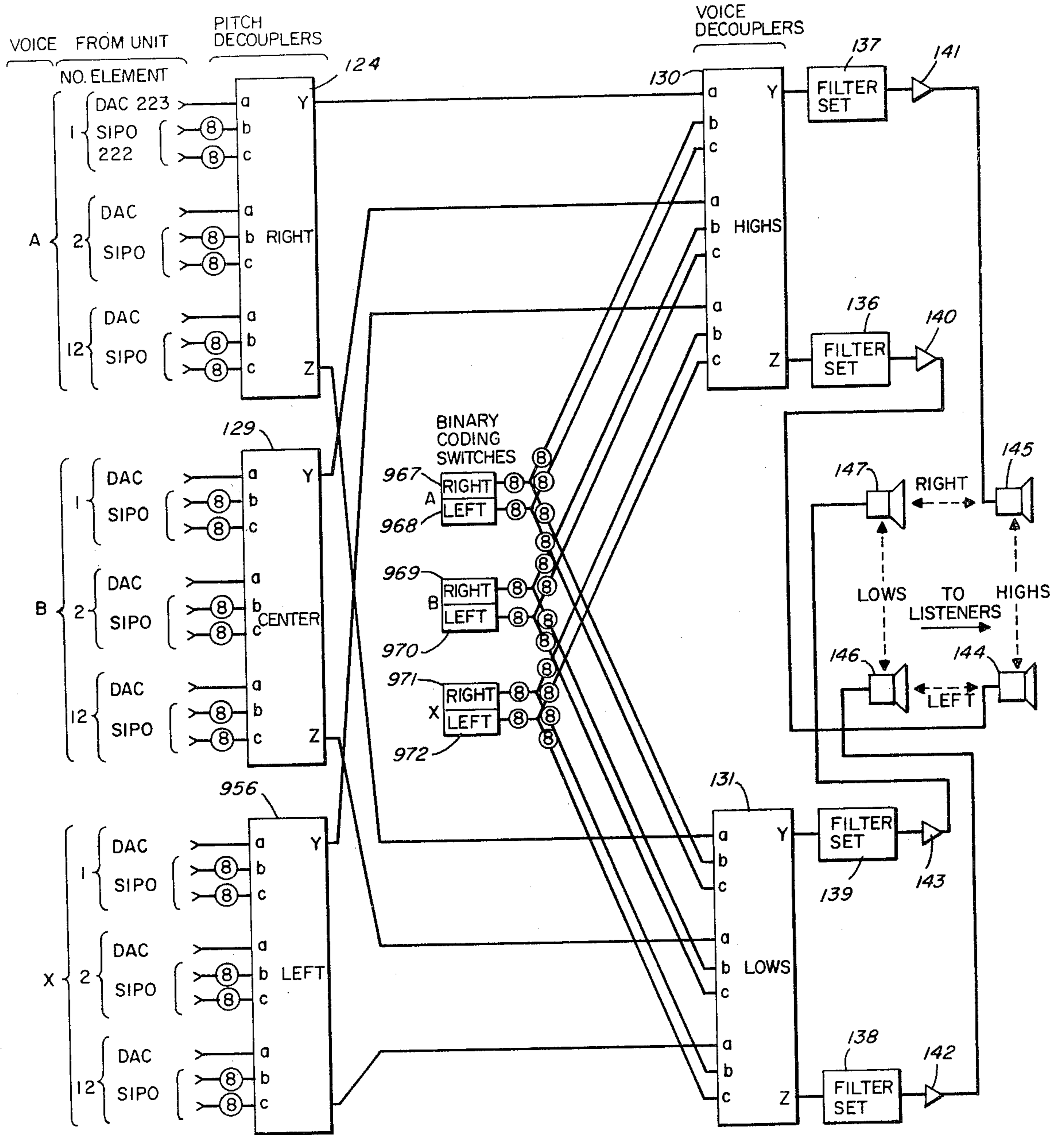
FIG. 10B
