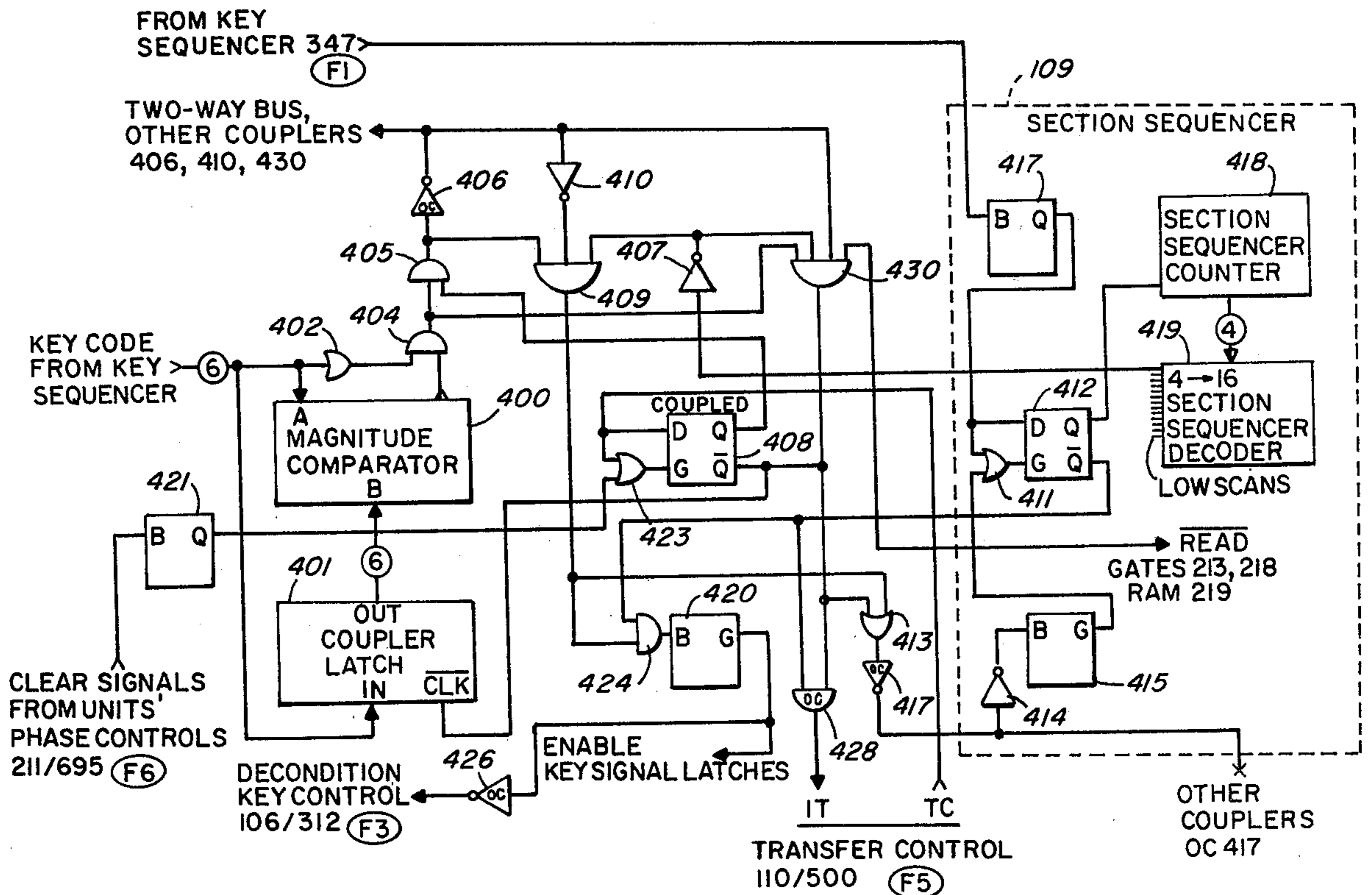
FIG. 4
