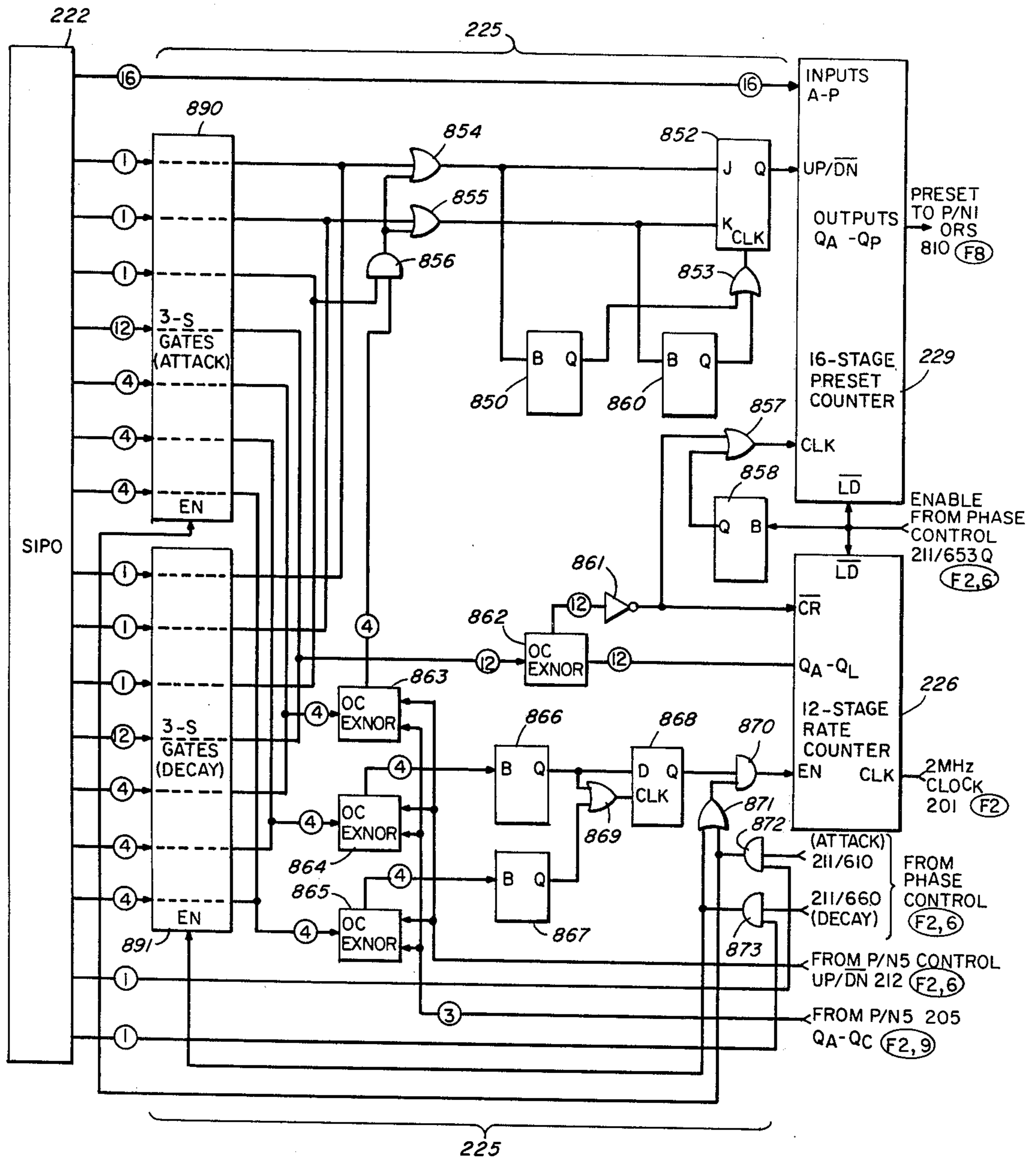
FIG. 14
