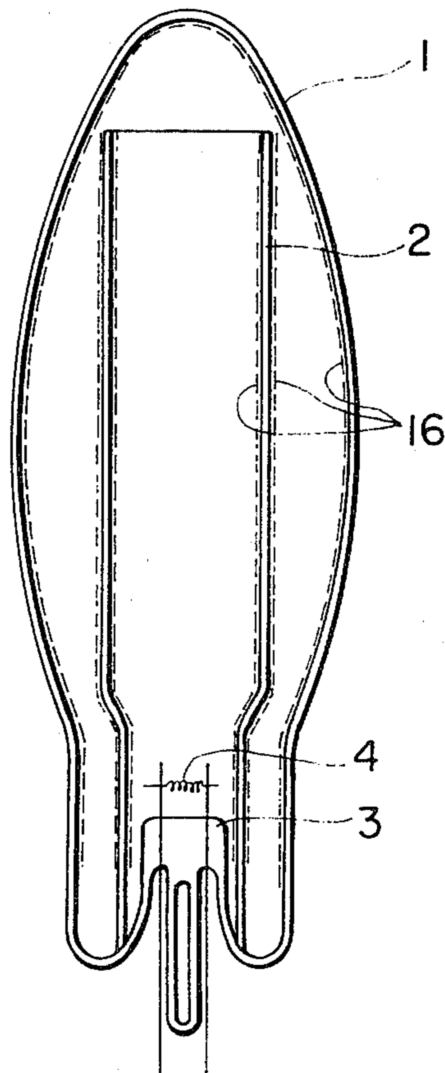
FIG. 10C
