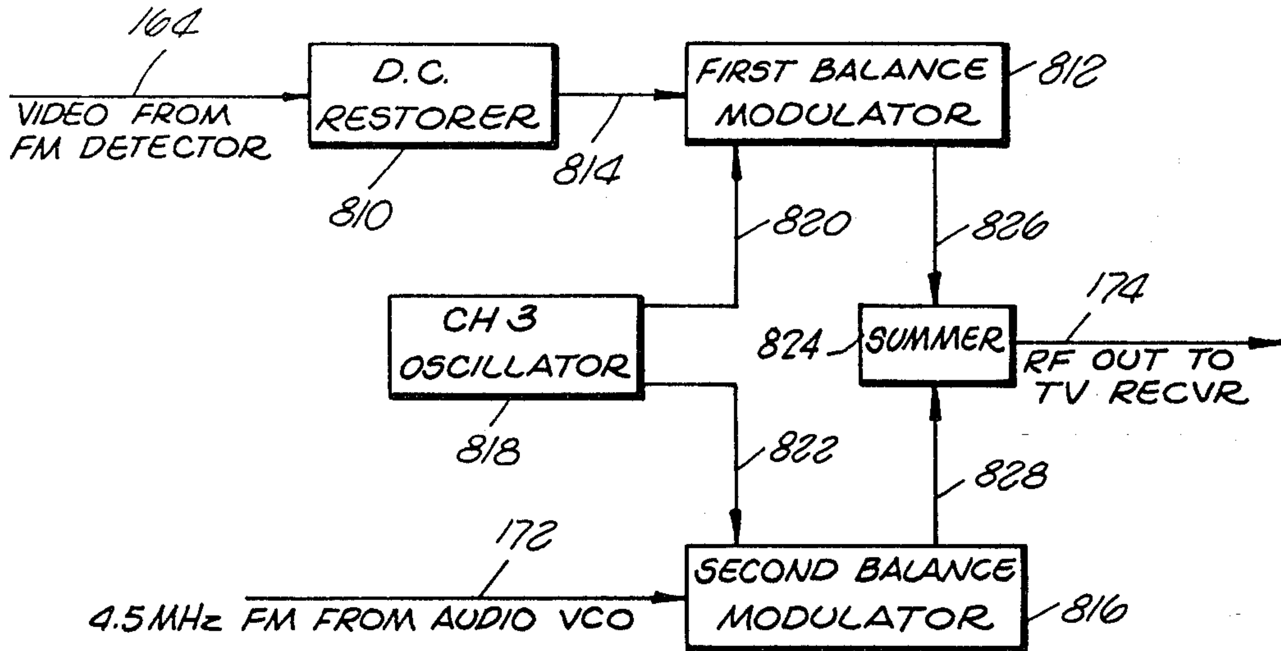
FIG. 24 RF MODULATOR
