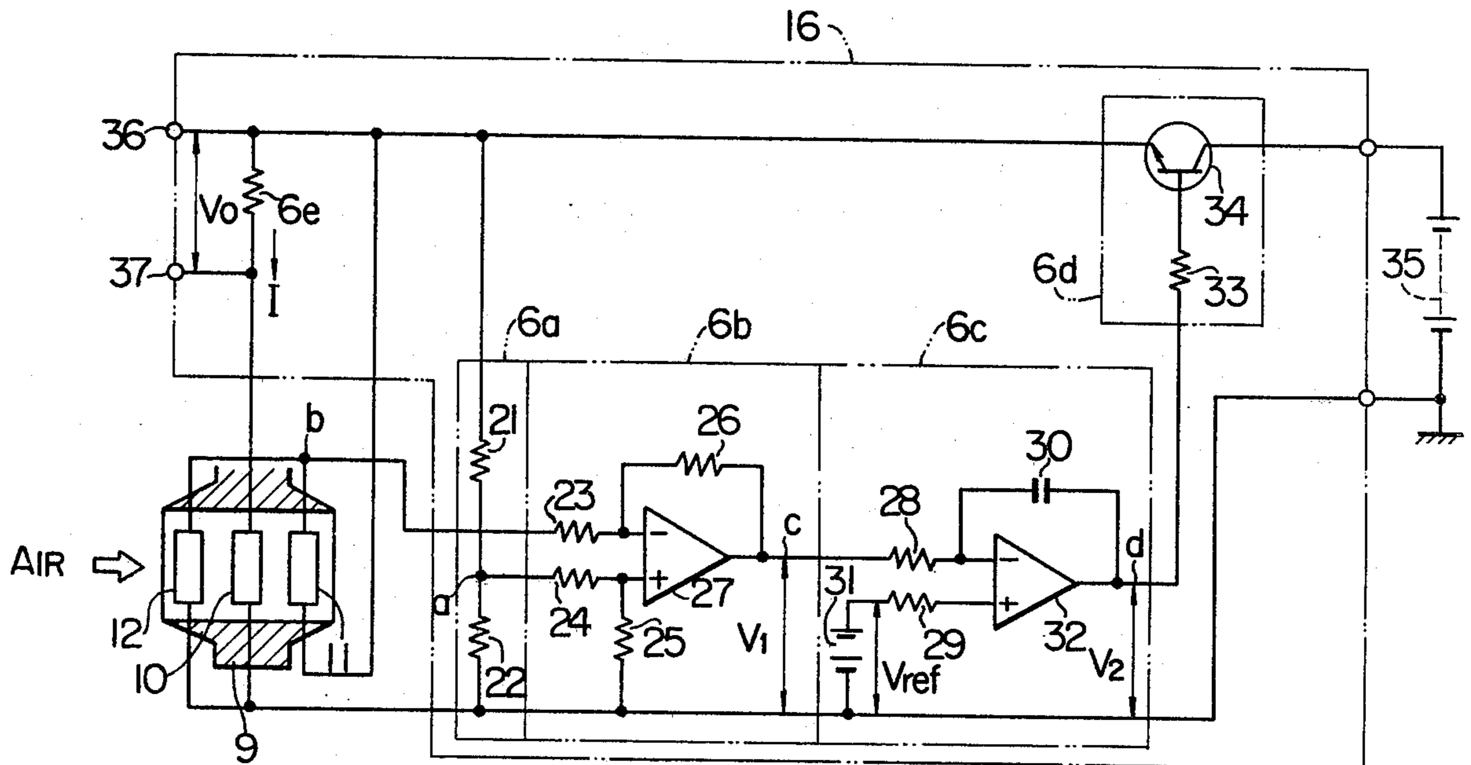
FIG. 7
