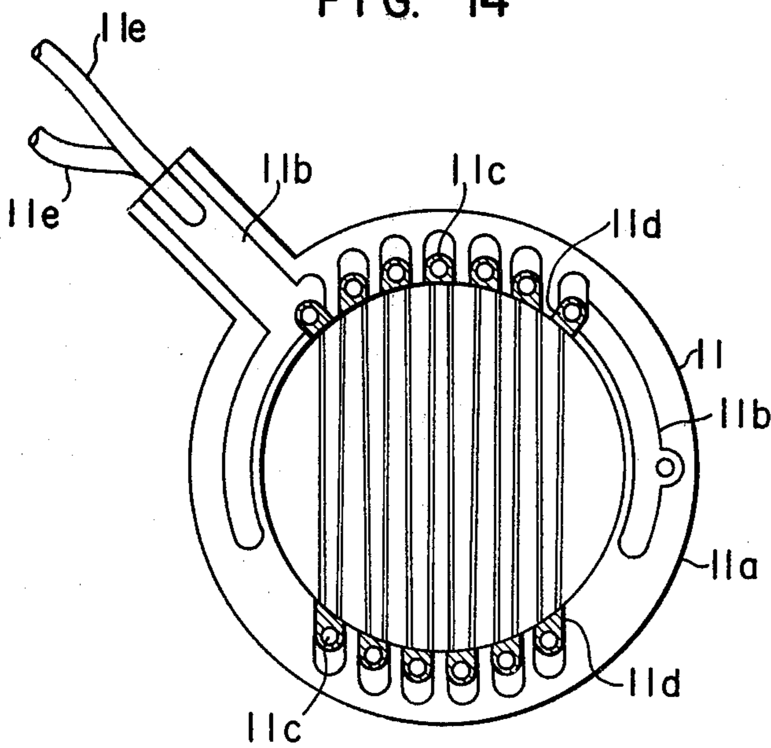
FIG. 14
