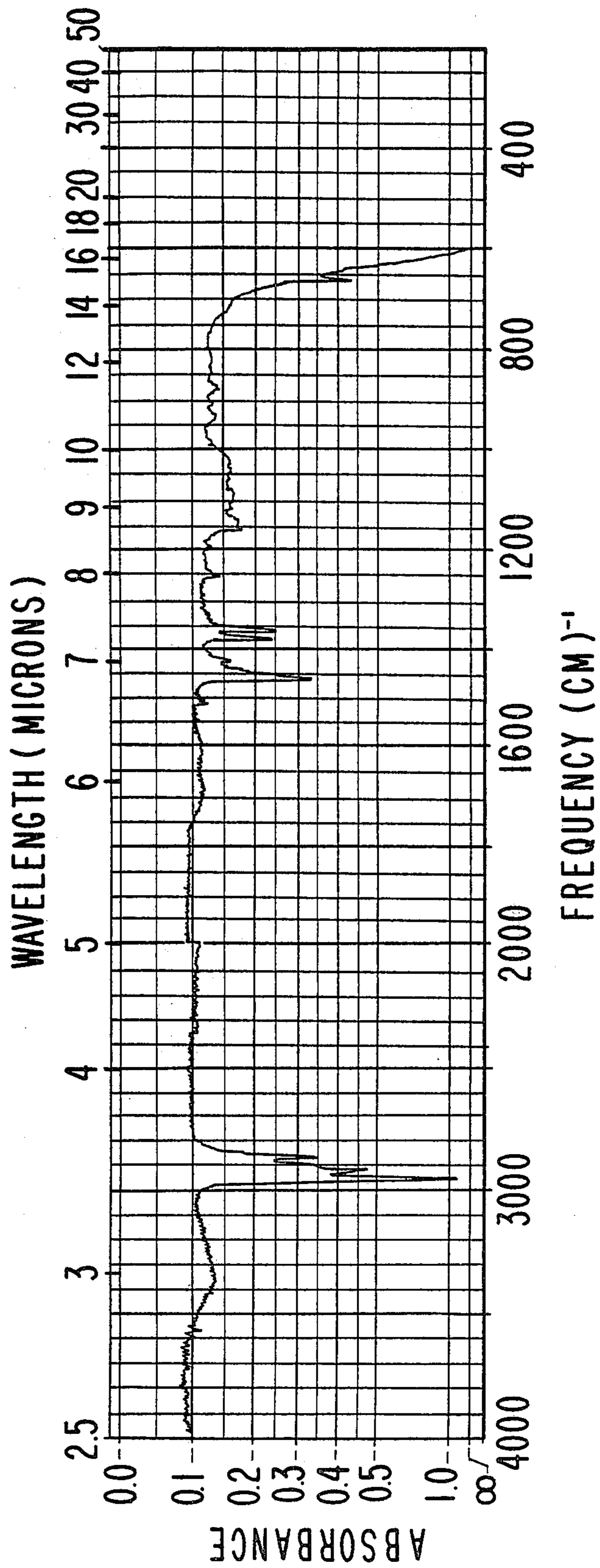
IR SPECTRUM, EXAMPLE I "CIS" ISOMER.
