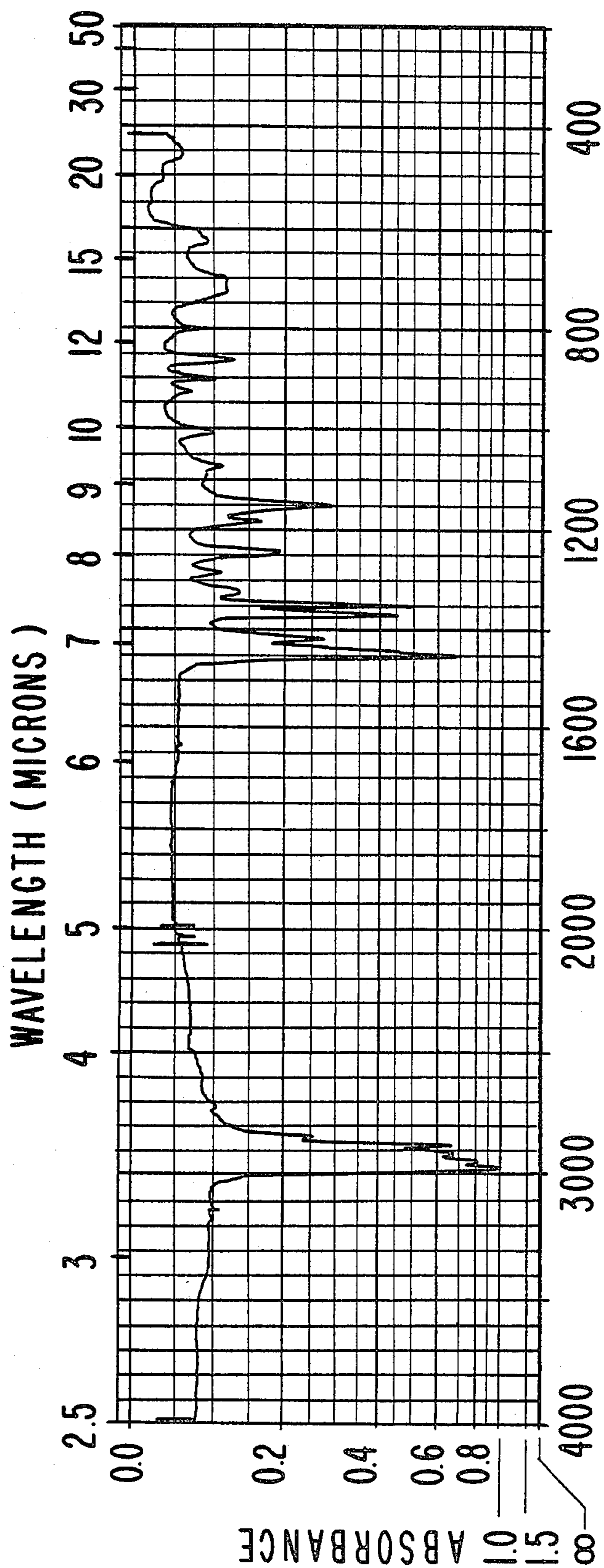
IR SPECTRUM, EXAMPLE I, FRACTION 5.
