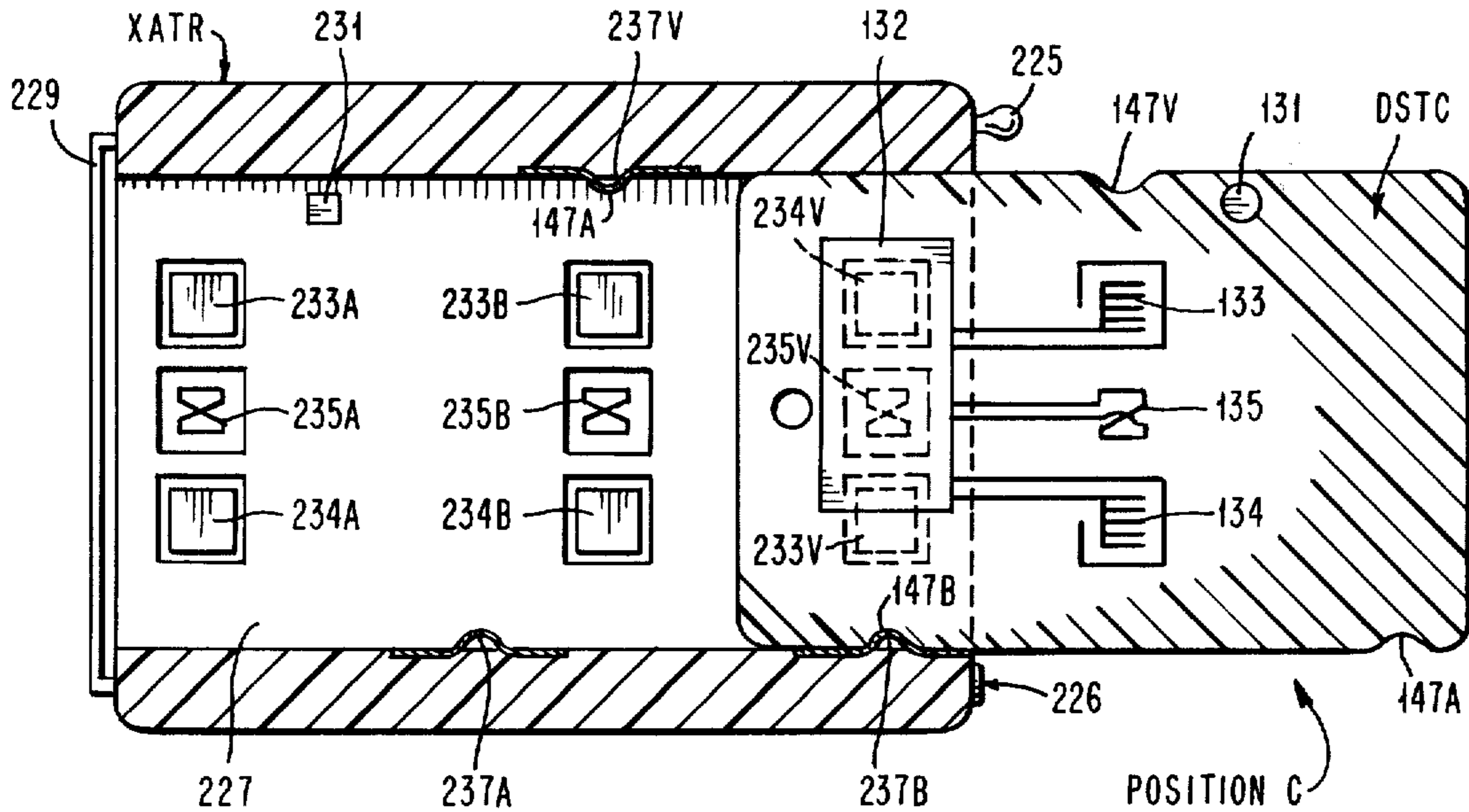
FIG. 8
