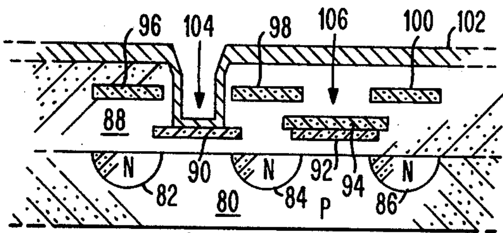
SECTION A-A'
