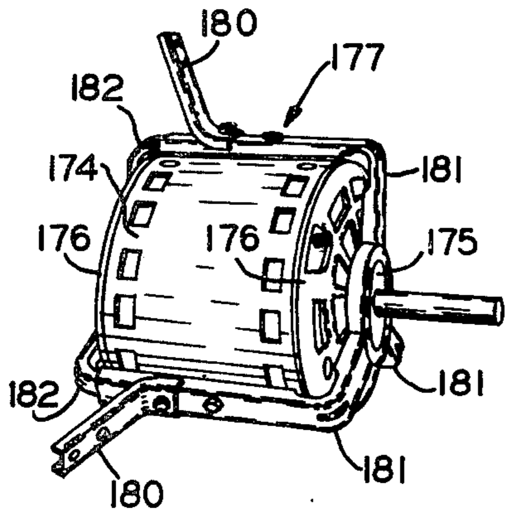
F I G. 27 PRIOR ART
