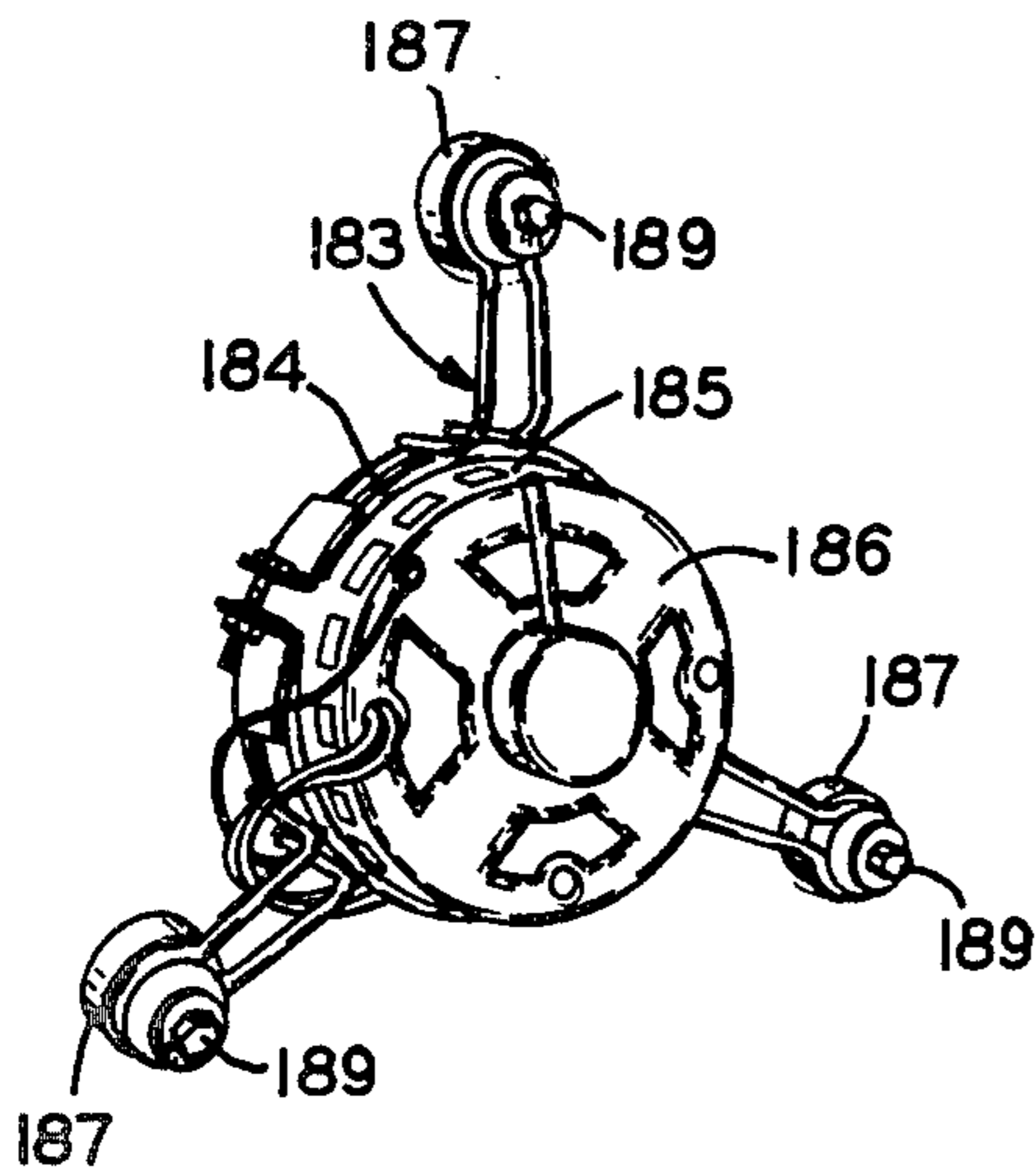
F I G. 25 PRIOR ART
