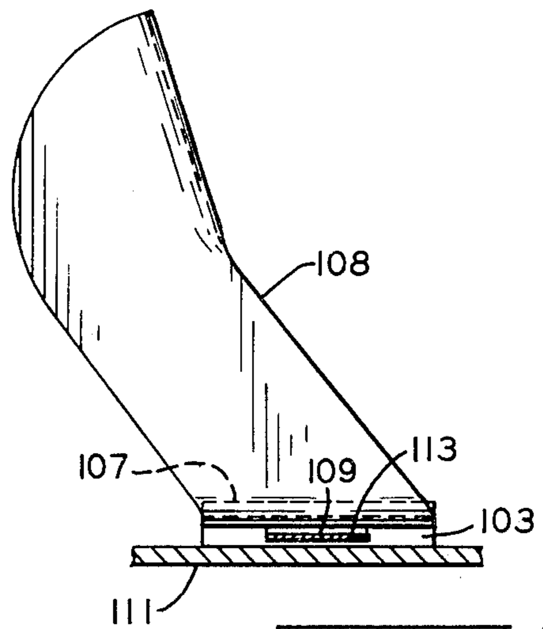
F I G. 16
