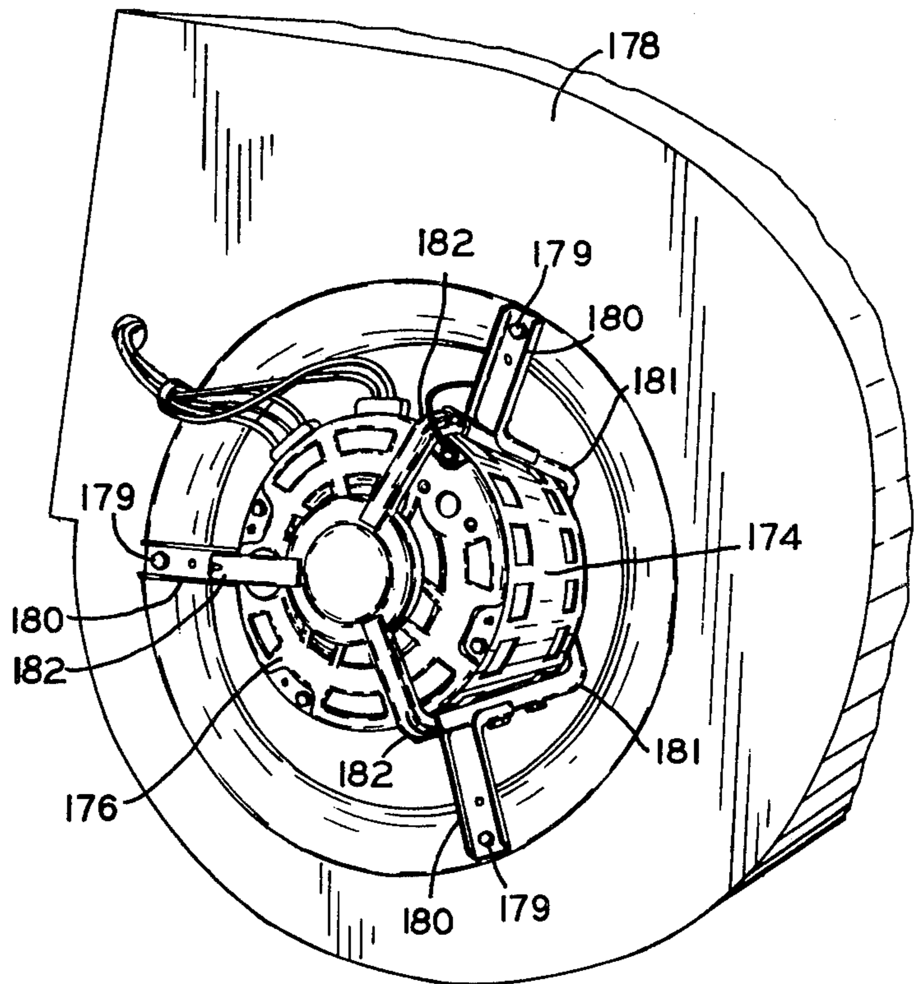
F I G. 28 PRIOR ART
