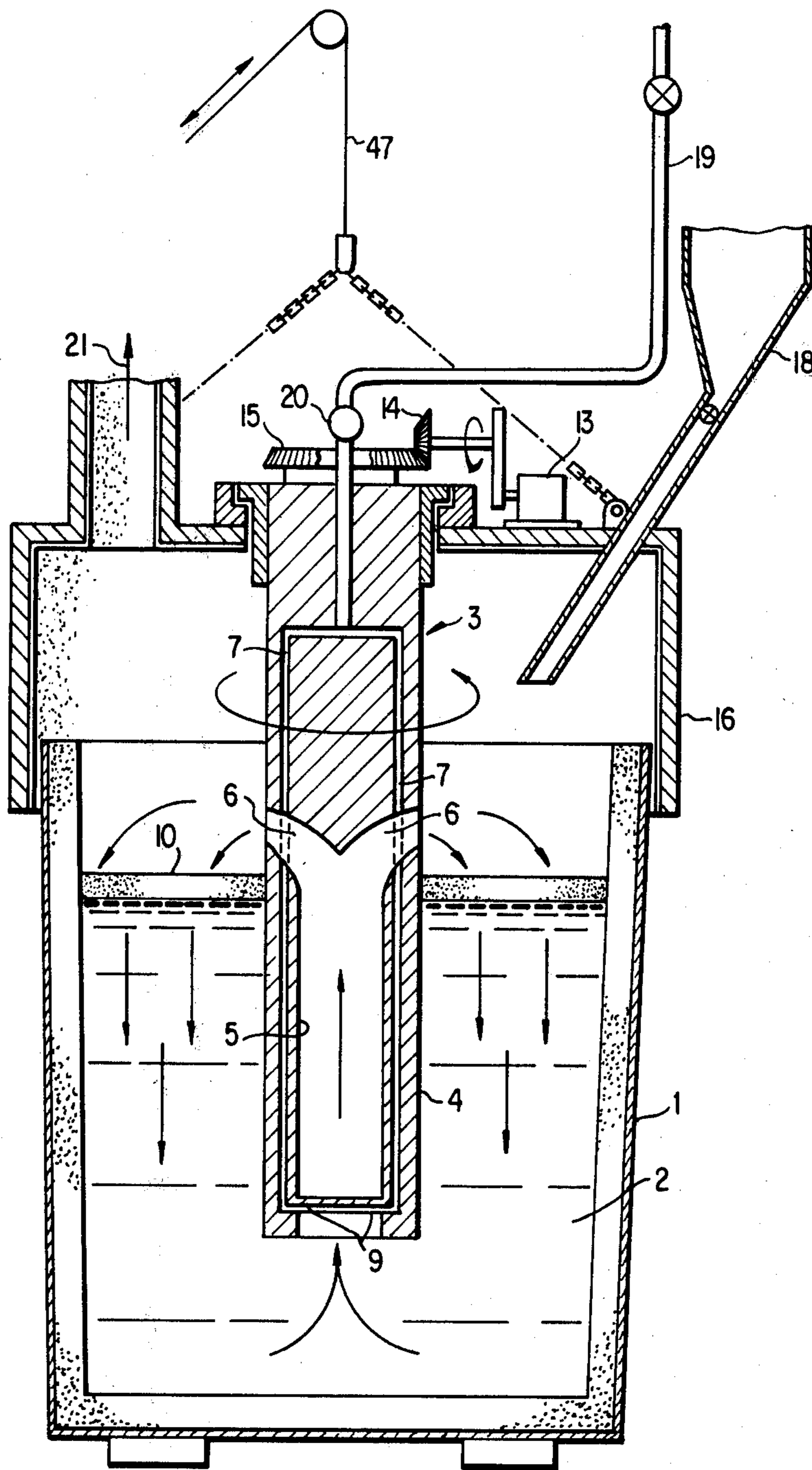
FIG. 8
