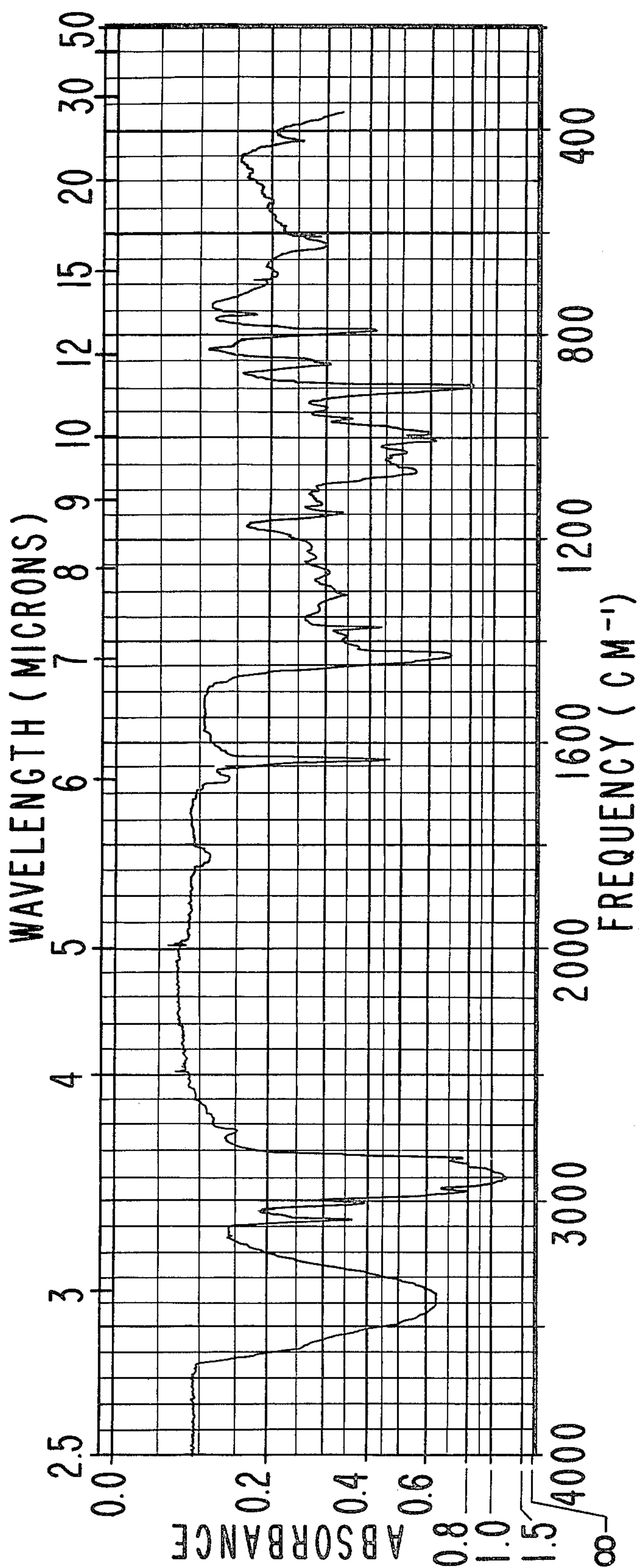
IR SPECTRUM FOR EXAMPLE V(A).
