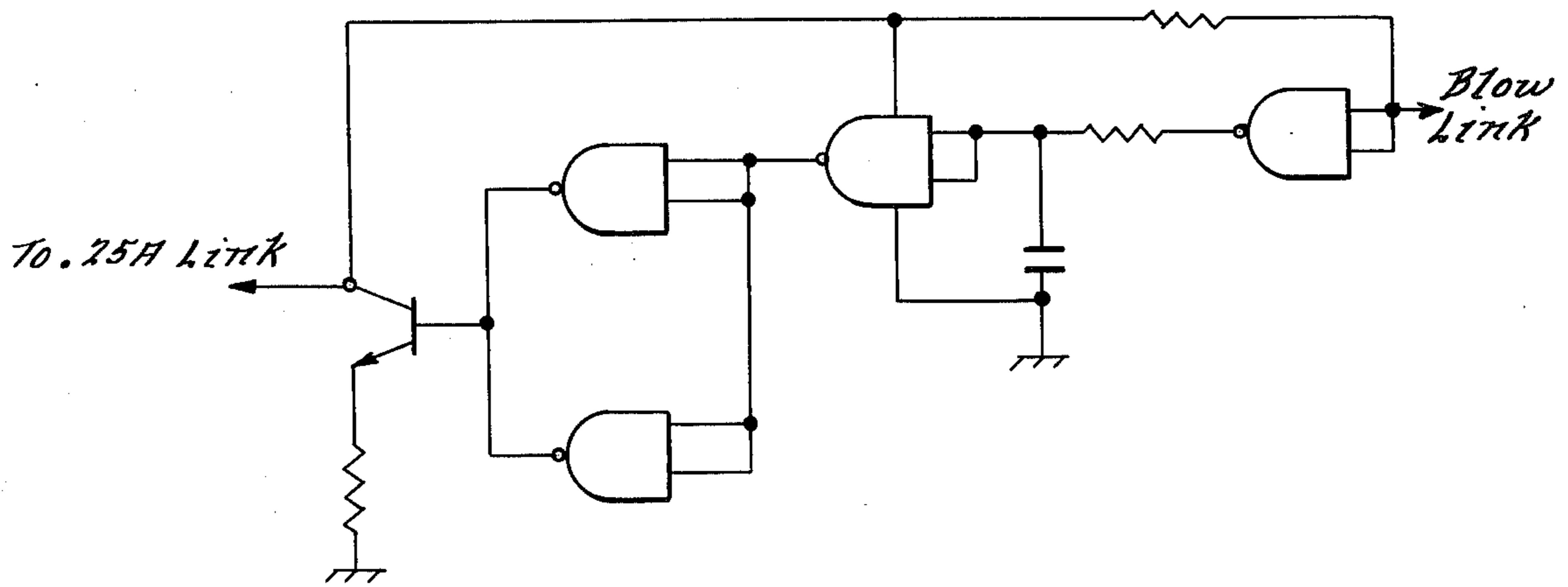
Link Blow Ckt.
