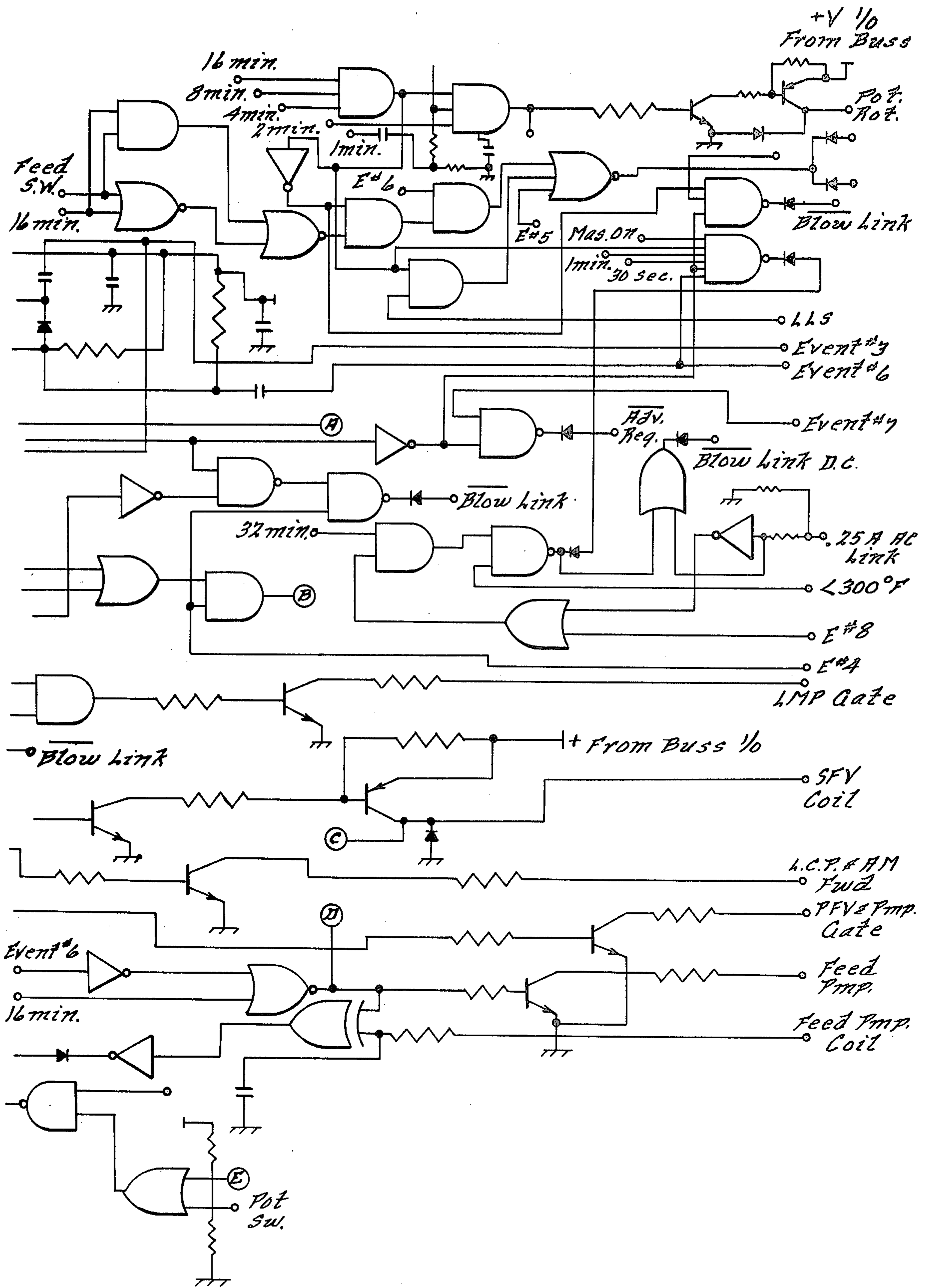
Logic & Timing Ckt. Fig. 26B.
