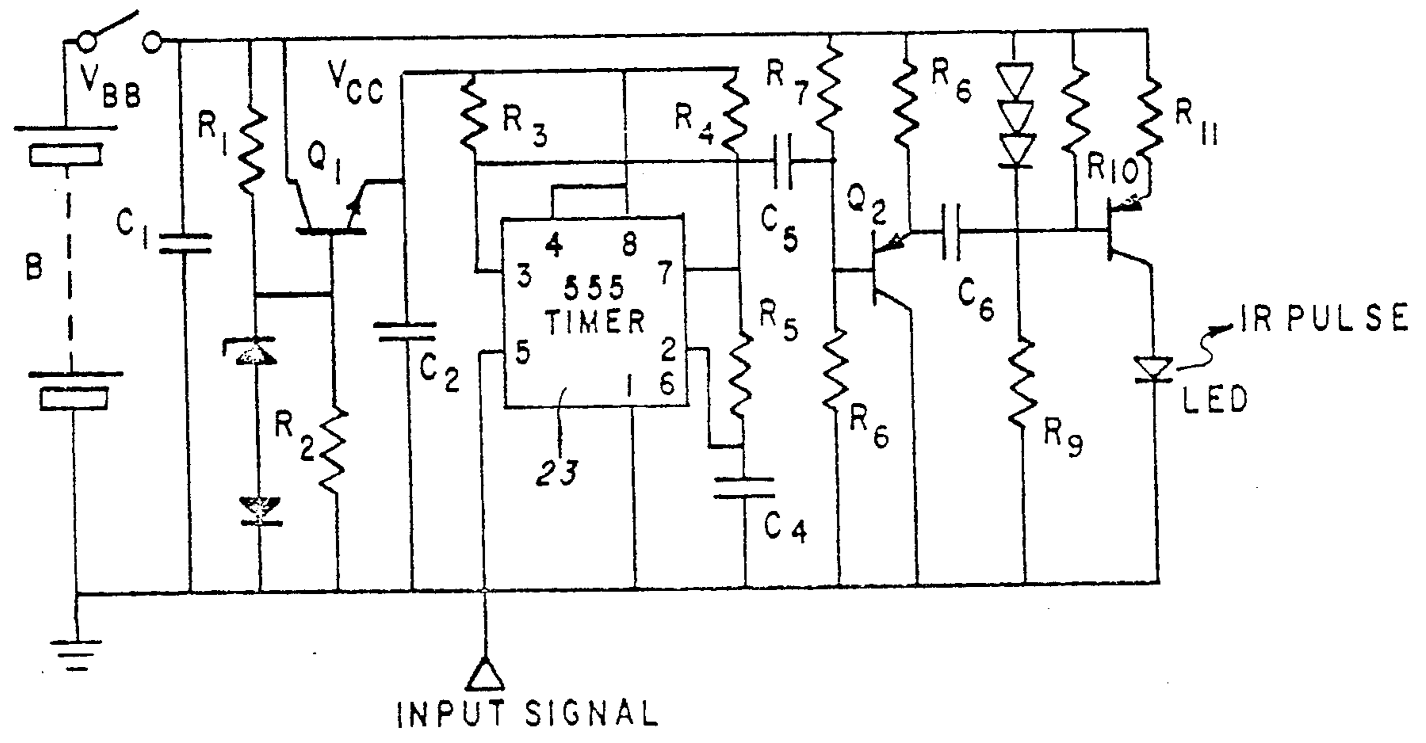
UNIVERSAL IR TRANSMITTER
