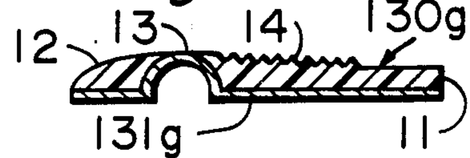
Fig. 13G
