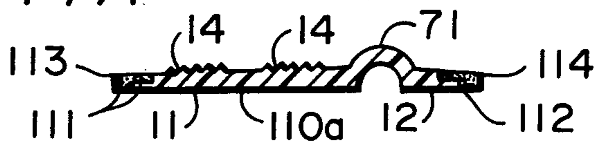
Fig. 11B
