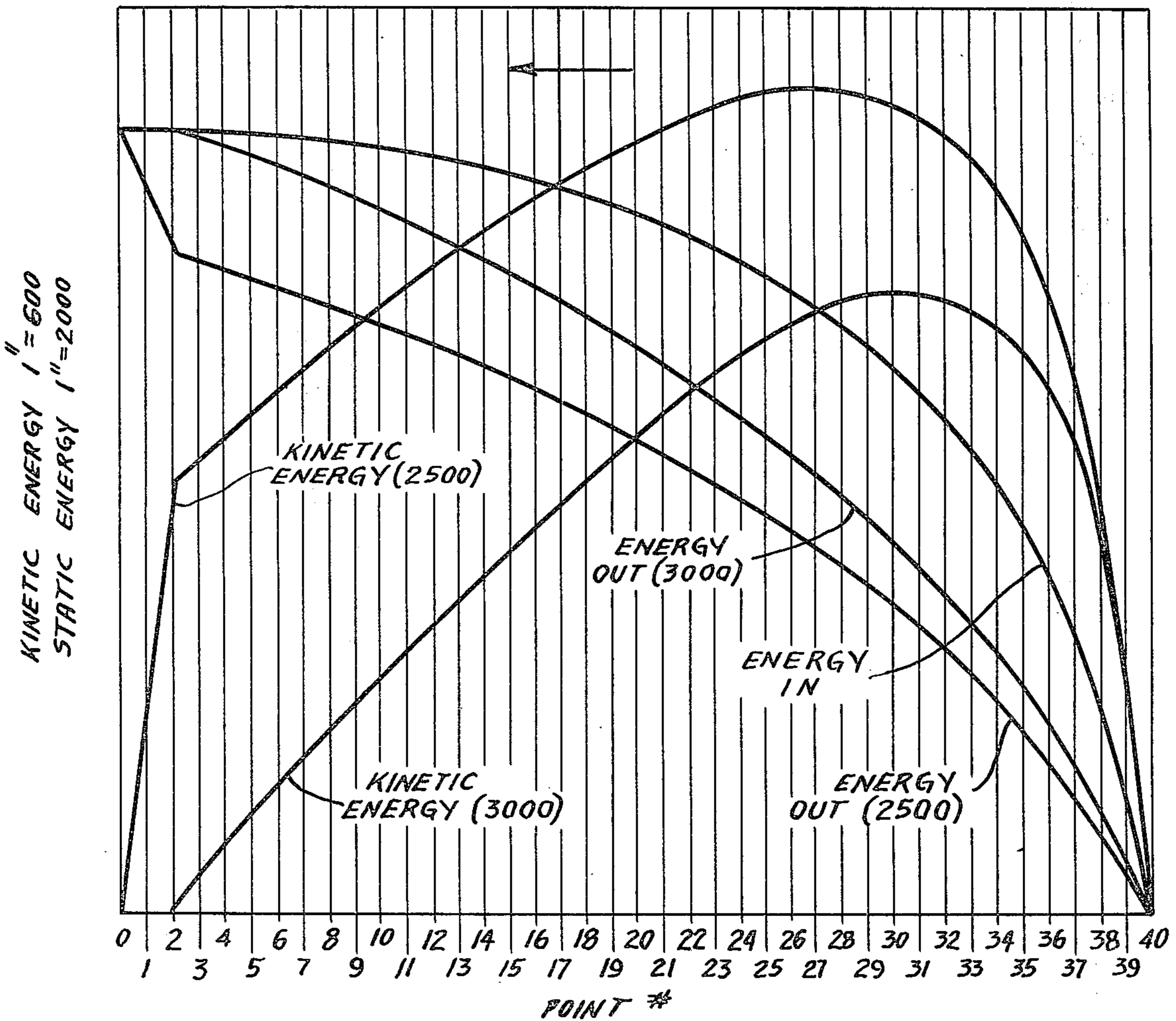
Fig. 12. COMBUSTION
