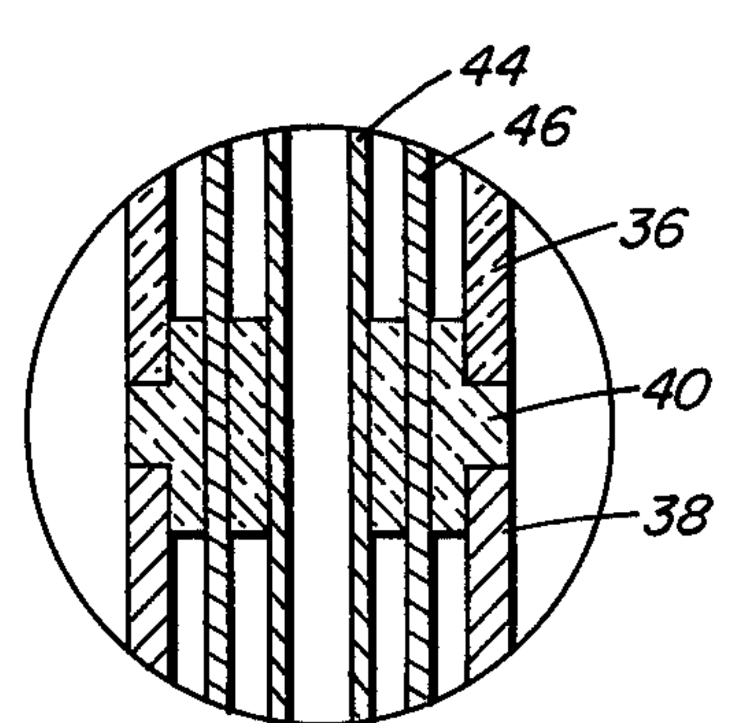
FIG. 2C
