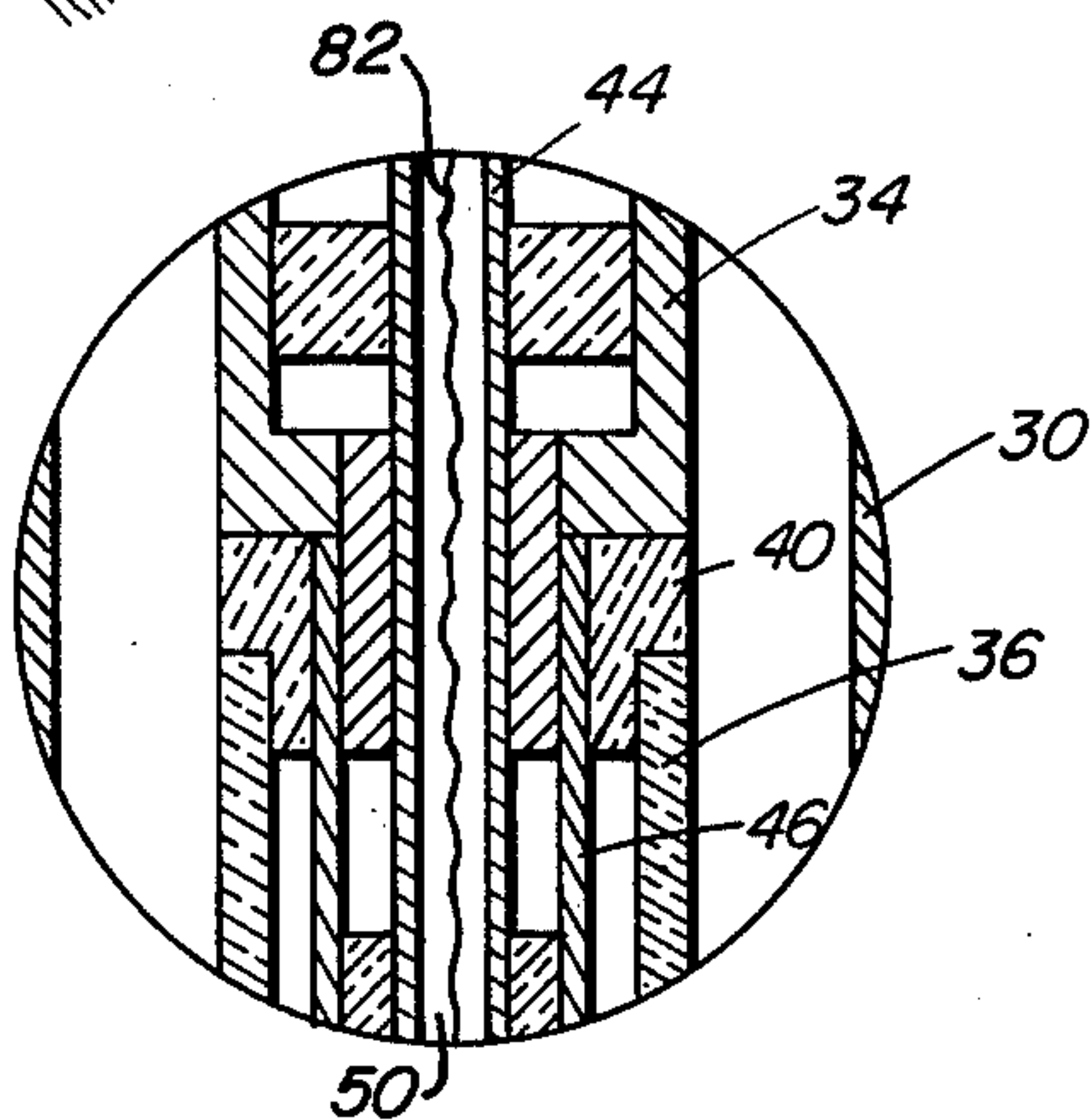
FIG. 2A
