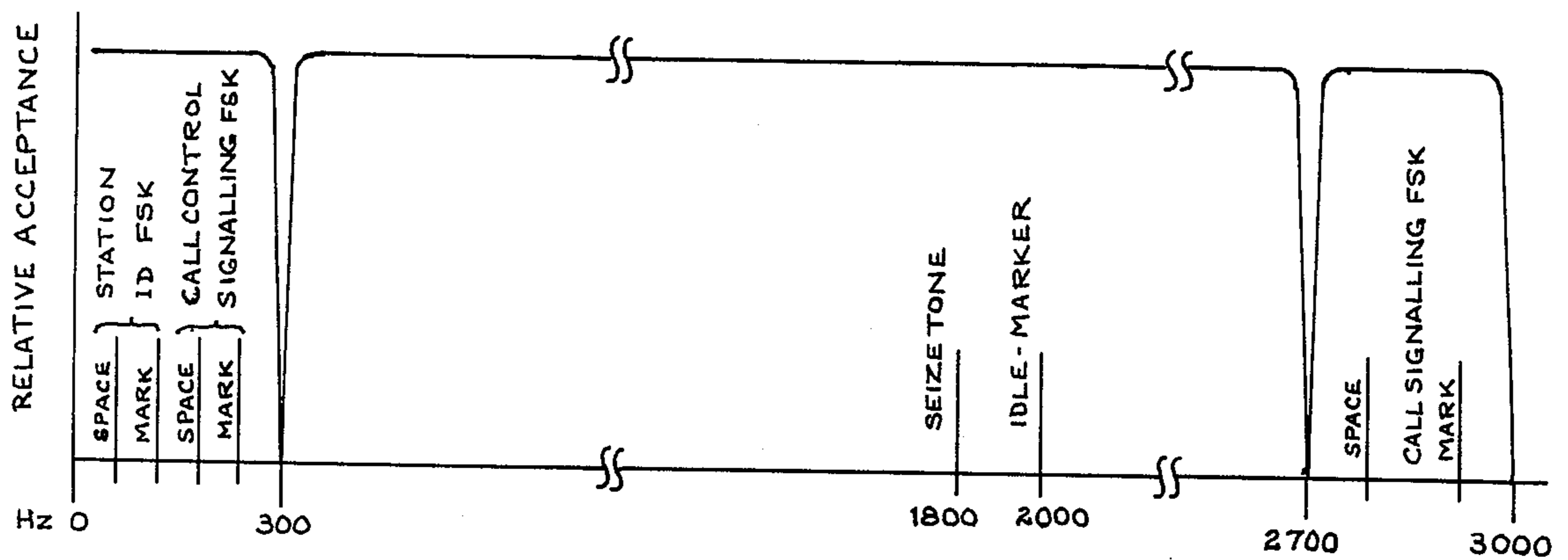
FIG. 1A. VF BASEBAND BASE-TO-MOBILE
