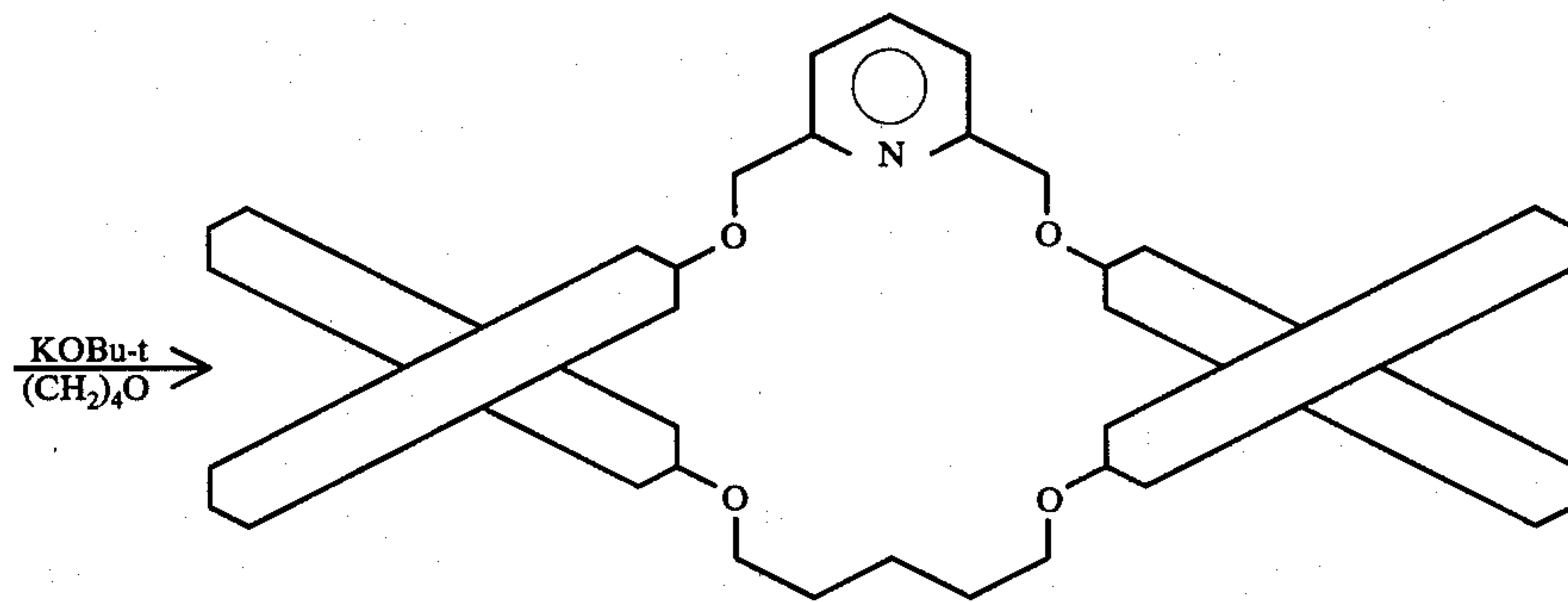
(SS)-23a
