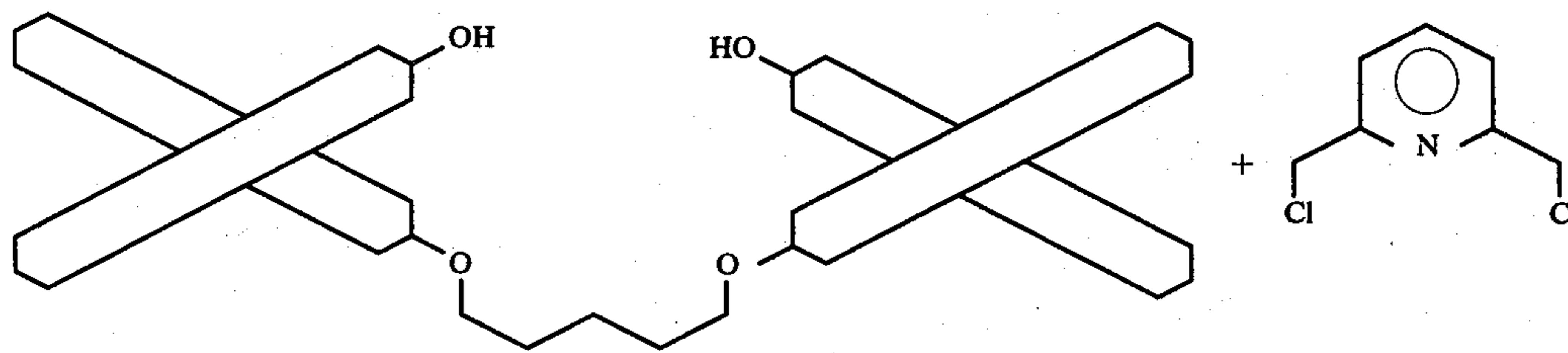
(SS)-22a
